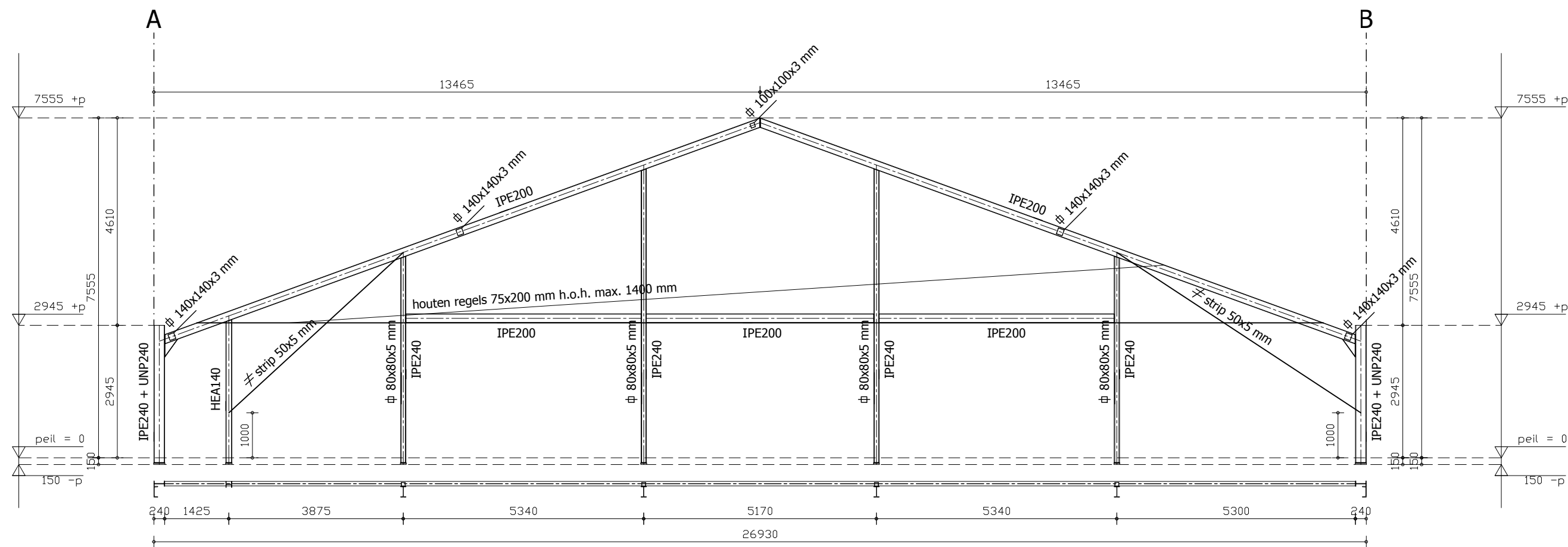
Spant 08 totaal 1x uitvoeren maten vooraf in het werk controleren hoogte maat incl. voetplaat en stelruimte spantverbindingen volgens berekeningen constructeur
