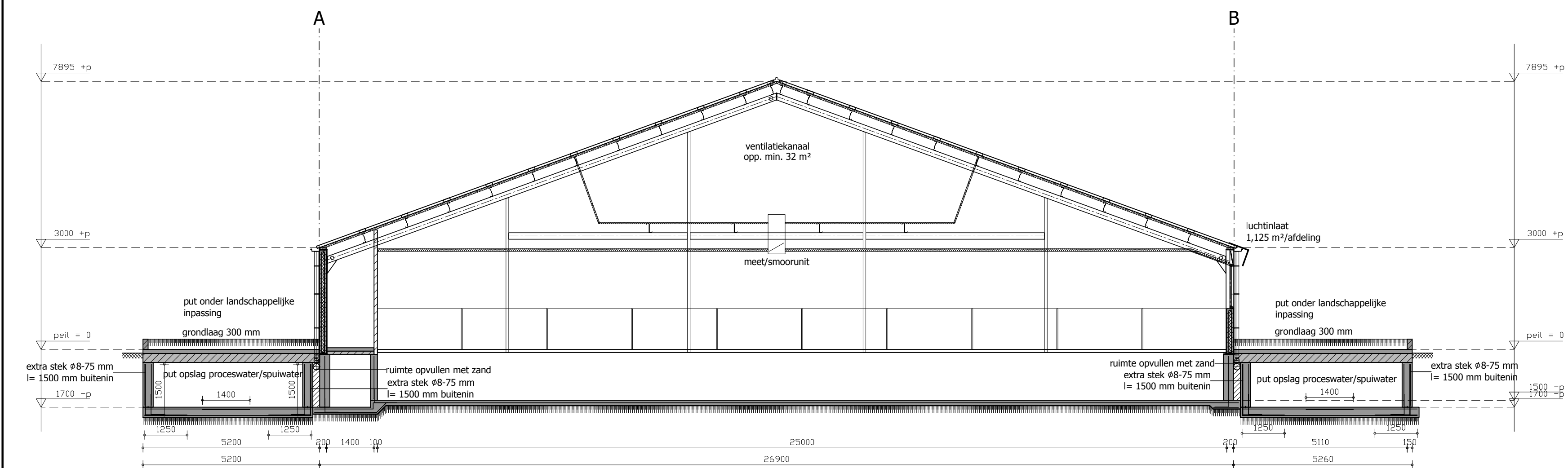
Doorsnede A-A
