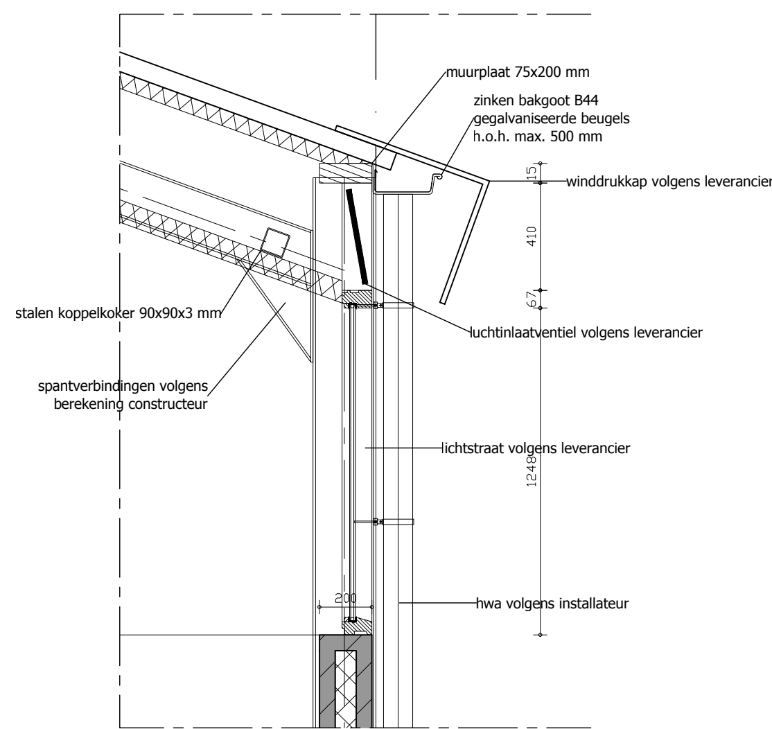
Detail lichtstraat
