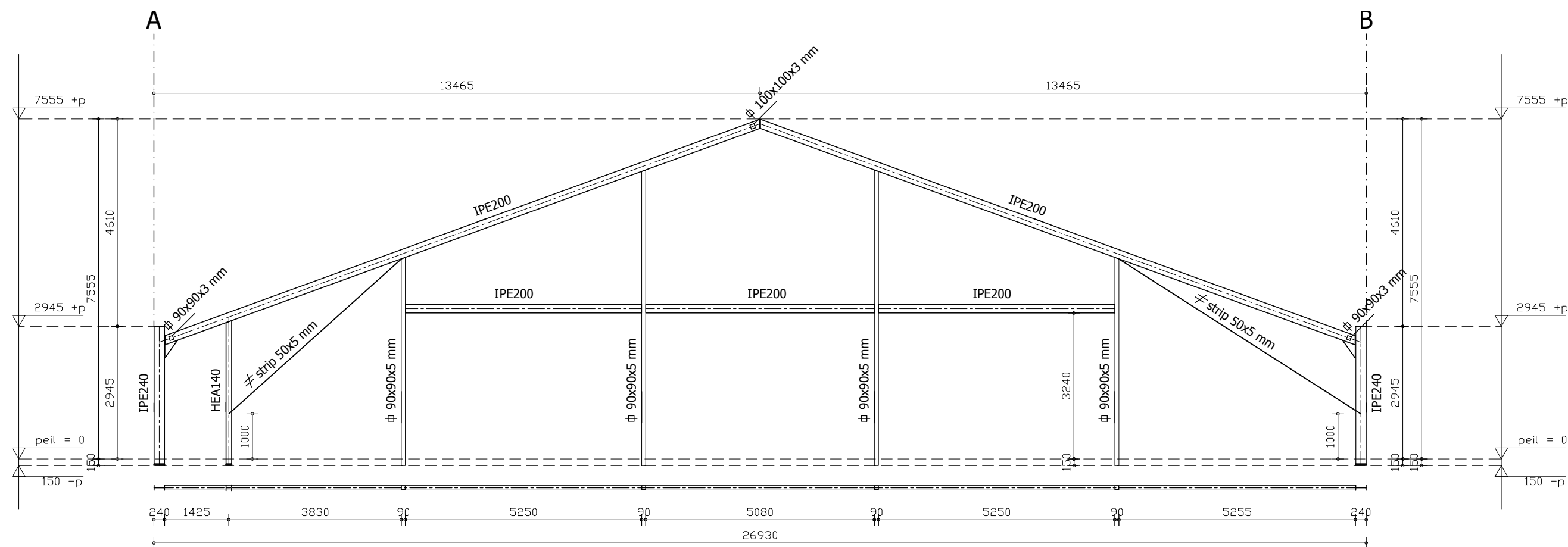
Spant 01 t/m 07 totaal 7x uitvoeren maten vooraf in het werk controleren hoogte maat incl. voetplaat en stelruimte spantverbindingen volgens berekeningen constructeur
