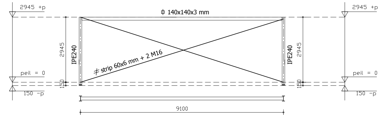
Windbok 1 totaal 6x uitvoeren maten vooraf in het werk controleren hoogte maat incl. voetplaat en stelruimte spantverbindingen volgens berekeningen constructeur
