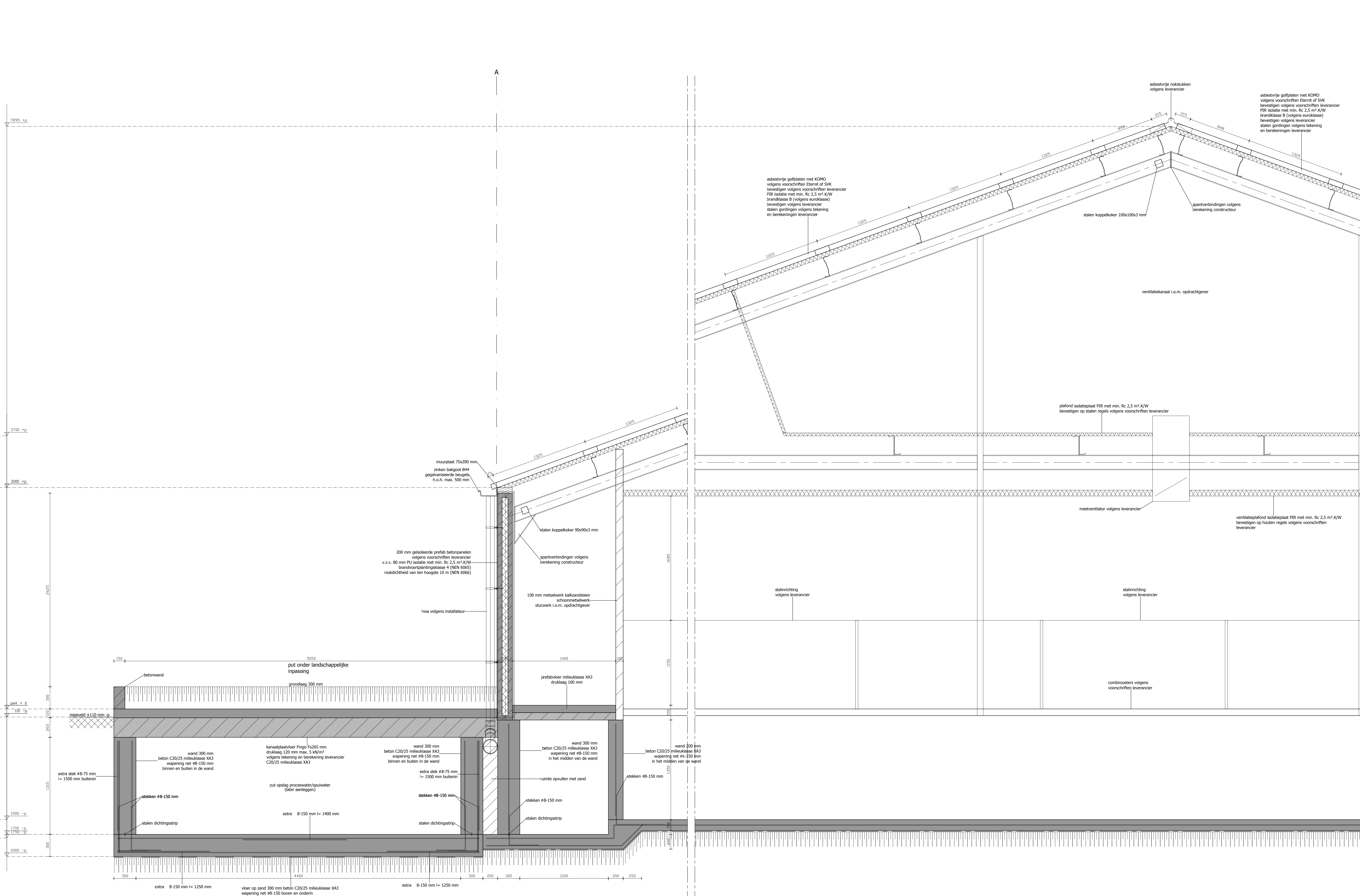
Doorsnede A-A
