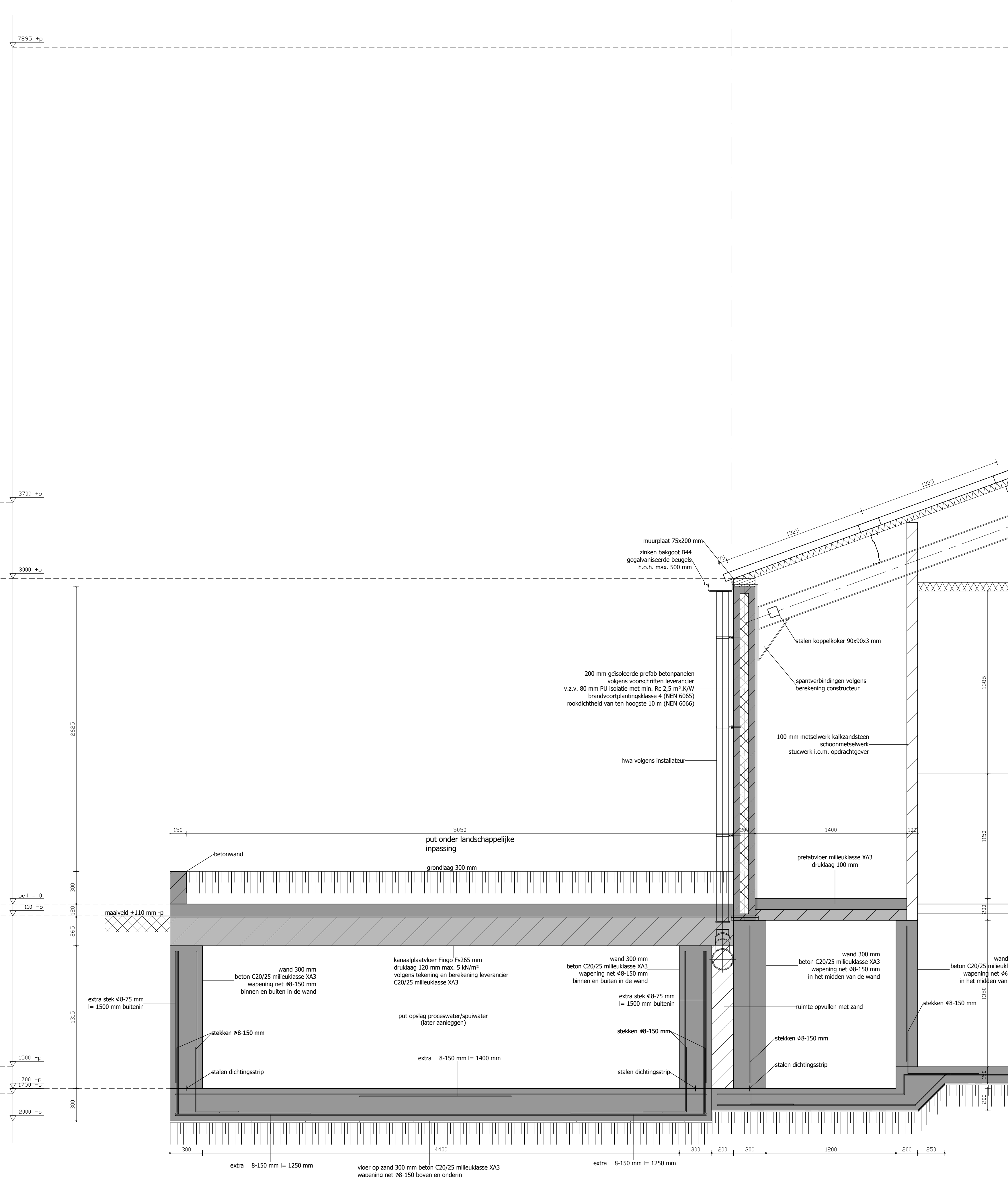
Doorsnede A-A
