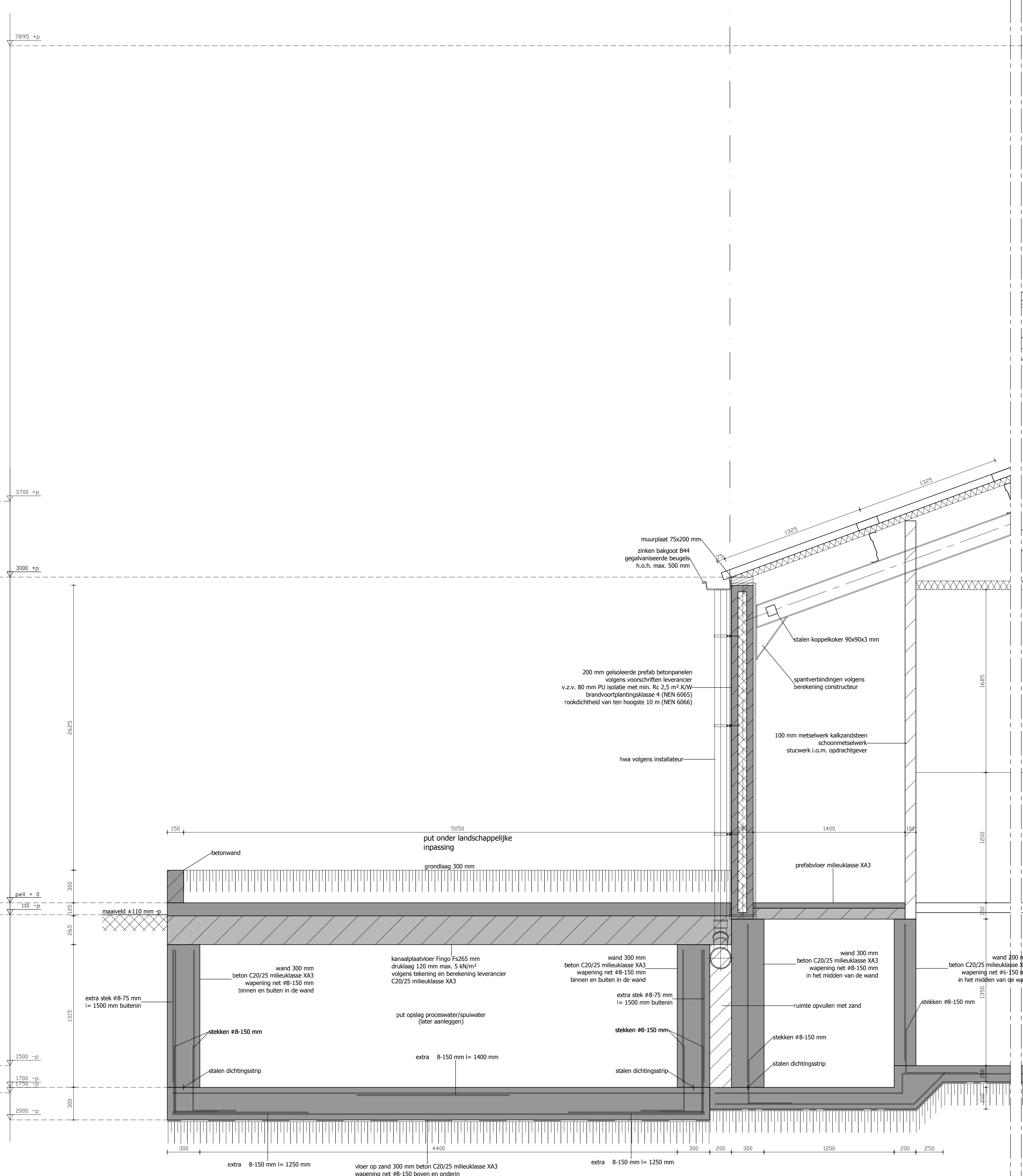
Doorsnede A-A
