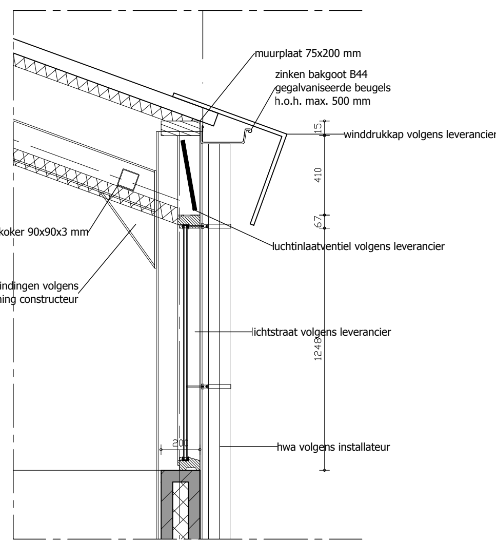
Detail lichtstraat
