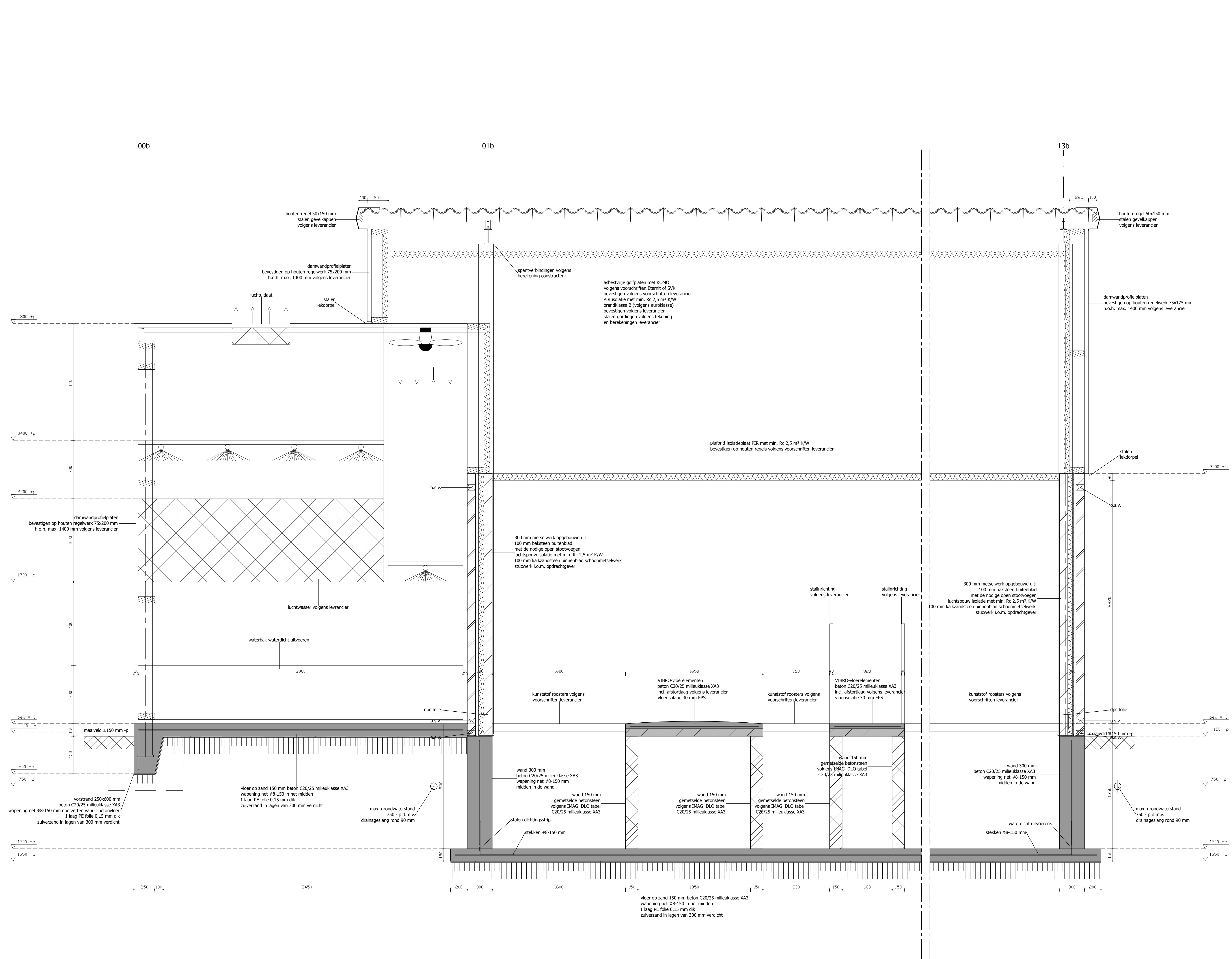
Doorsnede D-D
