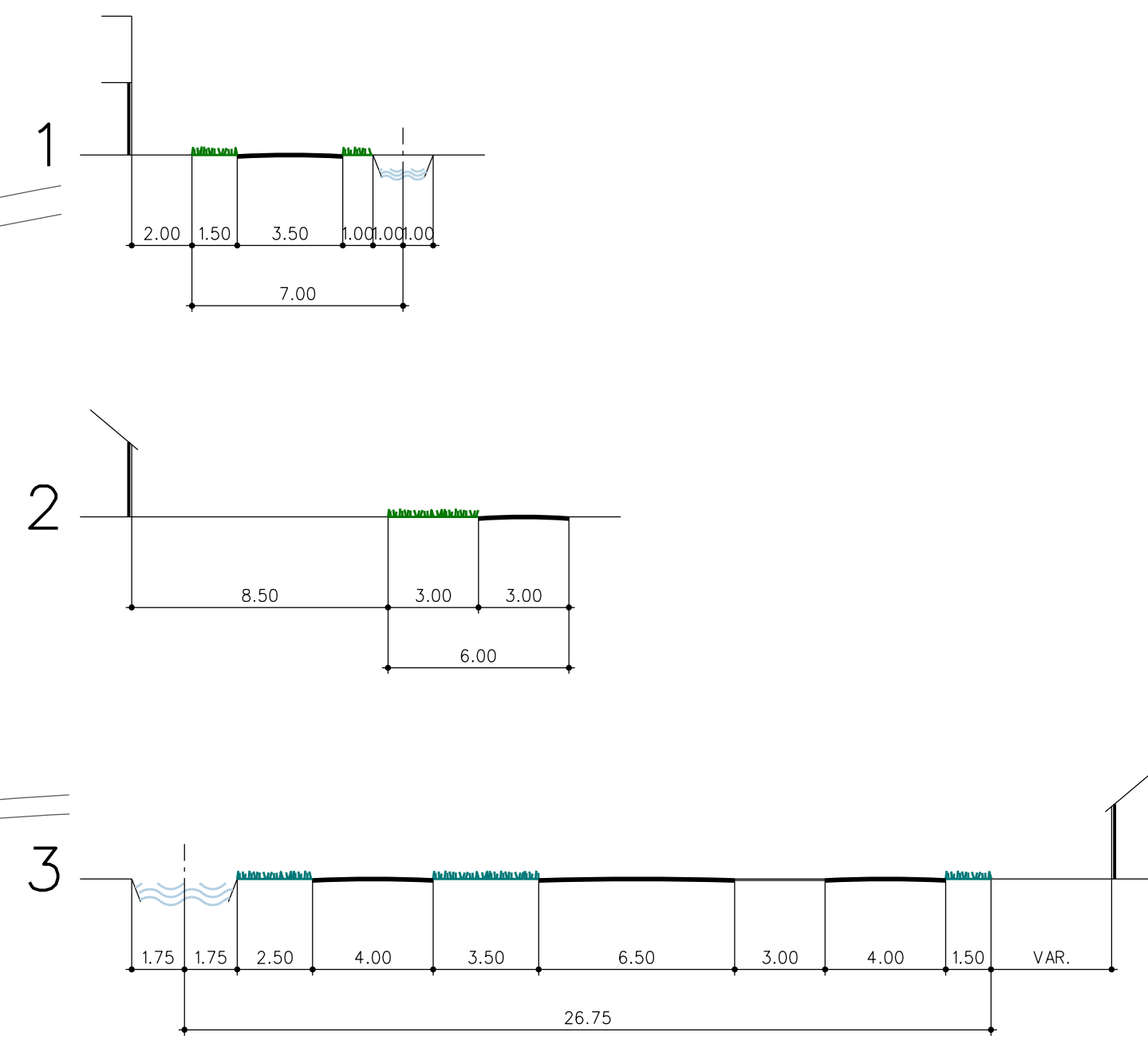
DWARSPROFIELEN SCHAAL 1:200
