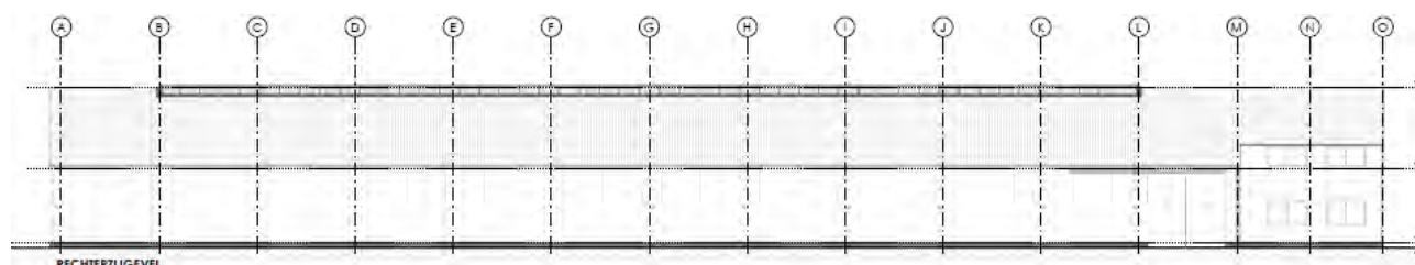
Figuur 3 | Aanzicht zijgevel
