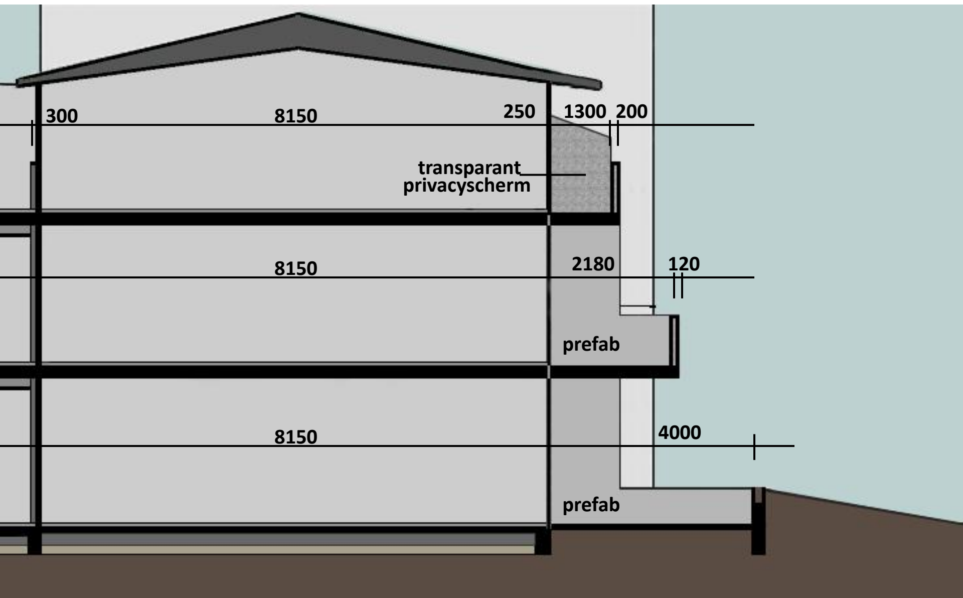
Doorsnede met afmetingen buitenruimtes
