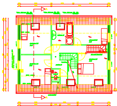
VERDIEPING
