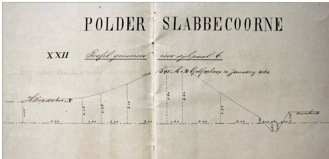
Afbeelding 17 Profiel van de zeedijk van de Slabbecoorpolder, 1871 (ZA RW, krt. 958).
