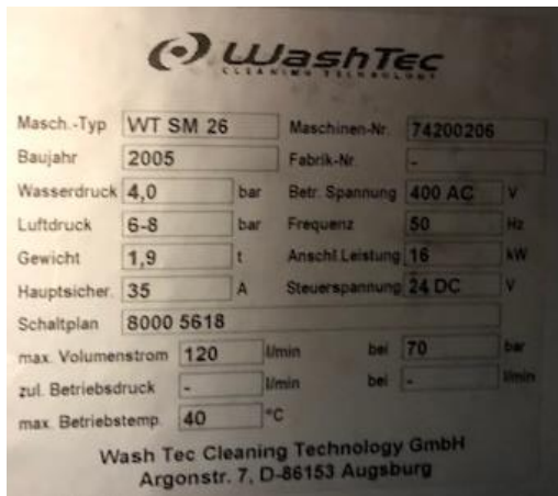
Afbeelding 3.1: Typeplaatse wasstraat (bron: FDarchitecten).
