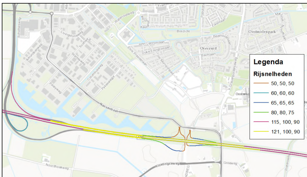
Figuur 7 Overzicht van de gehanteerde rijsnelheden in de geluidsberekeningen
