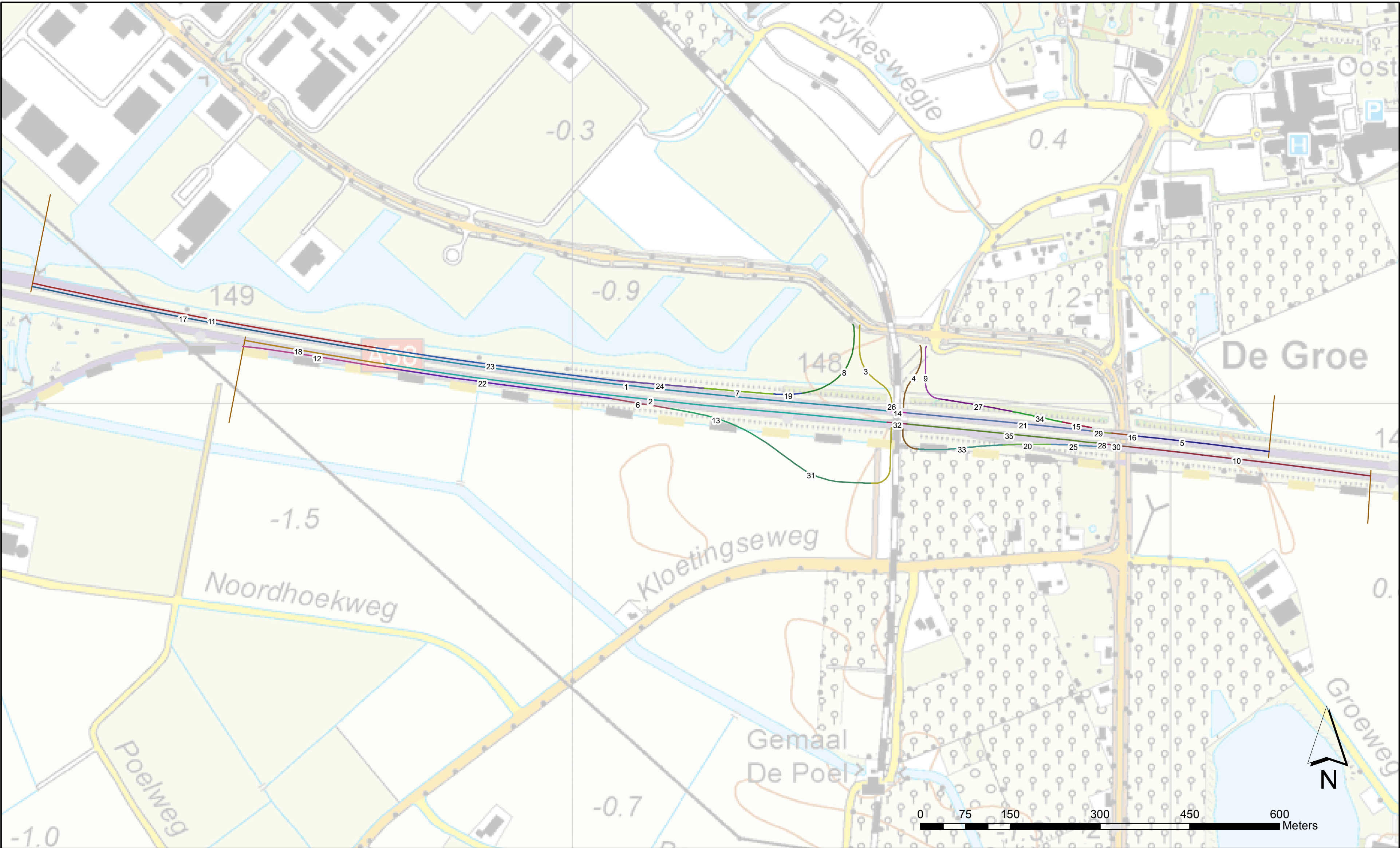
Figuur 1: Wegvaknummering
