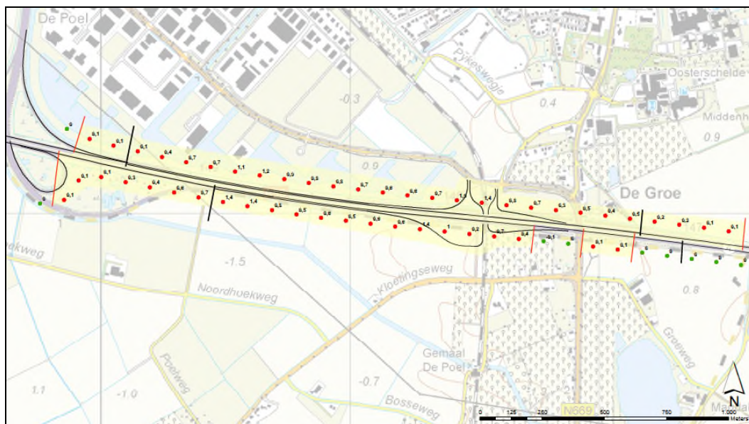
Figuur 8 Ligging project (zwarte lijn) en onderzoeksgebied (rode lijn) zuidwestzijde tot waar de geluidproductieplafonds worden overschreden wanneer geen maatregelen worden getroffen.
