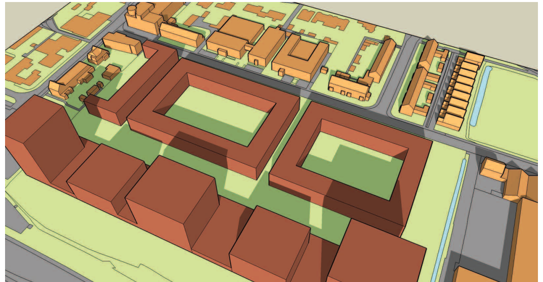
nieuwe planologische situatie 21 september 11:00
