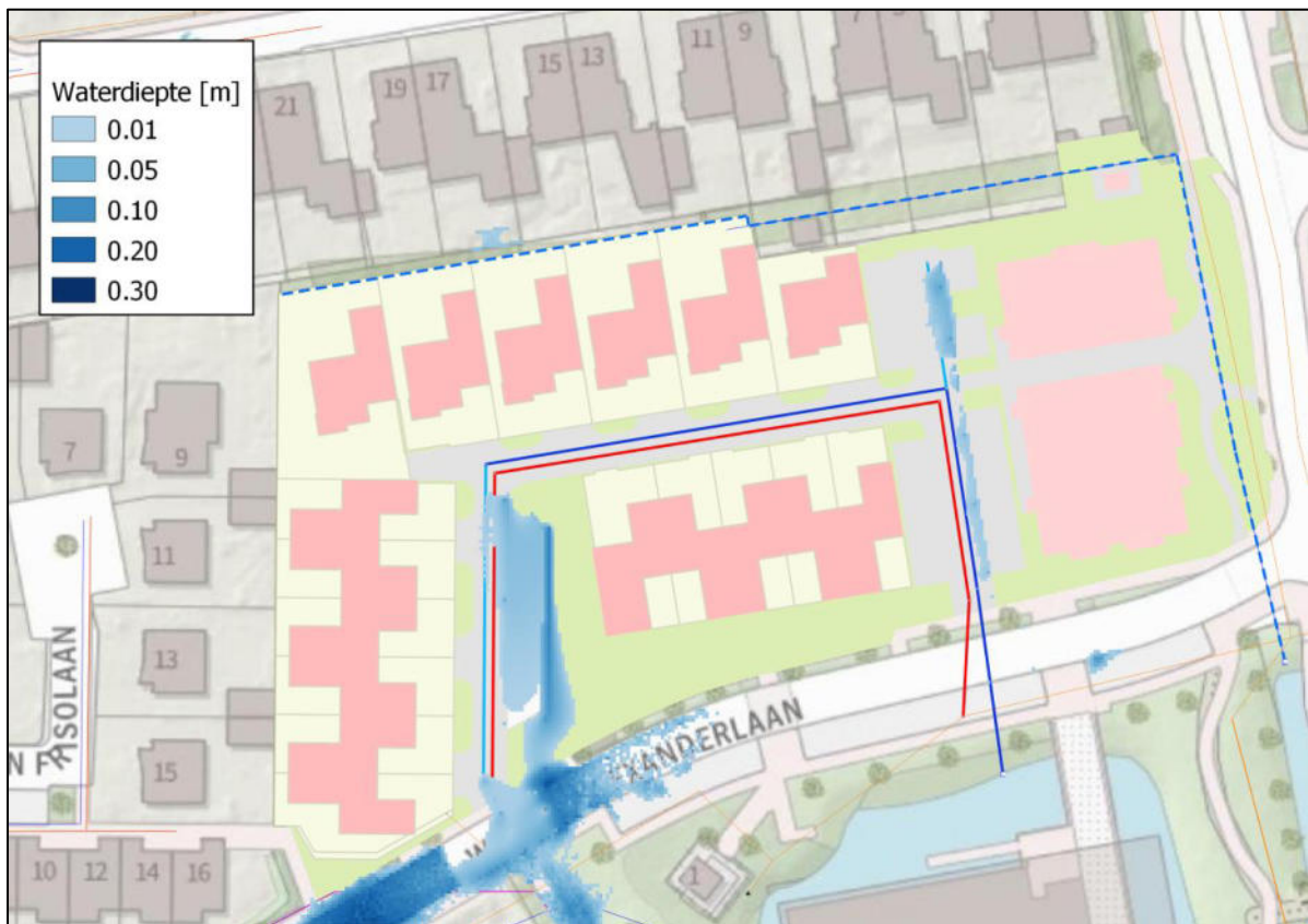
Afbeelding 3-10: Stresstest 90 mm/h
