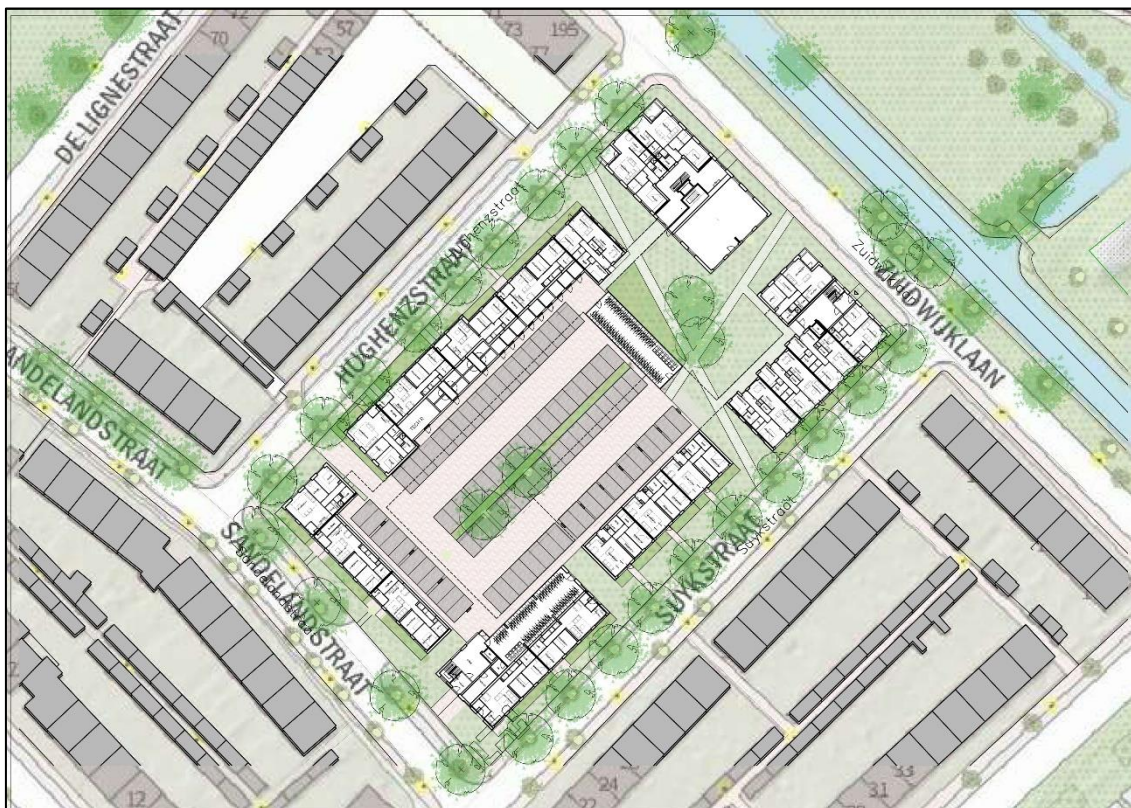
Figuur 9: Bovenaanzicht toekomstige situatie - Studio VVKH
