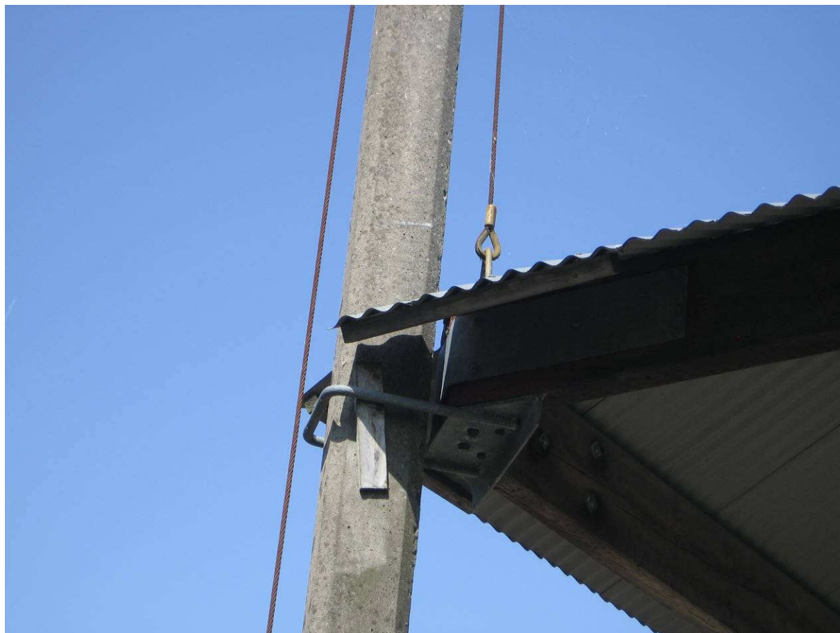
5. Oude toestand kolom en hefwerk.
