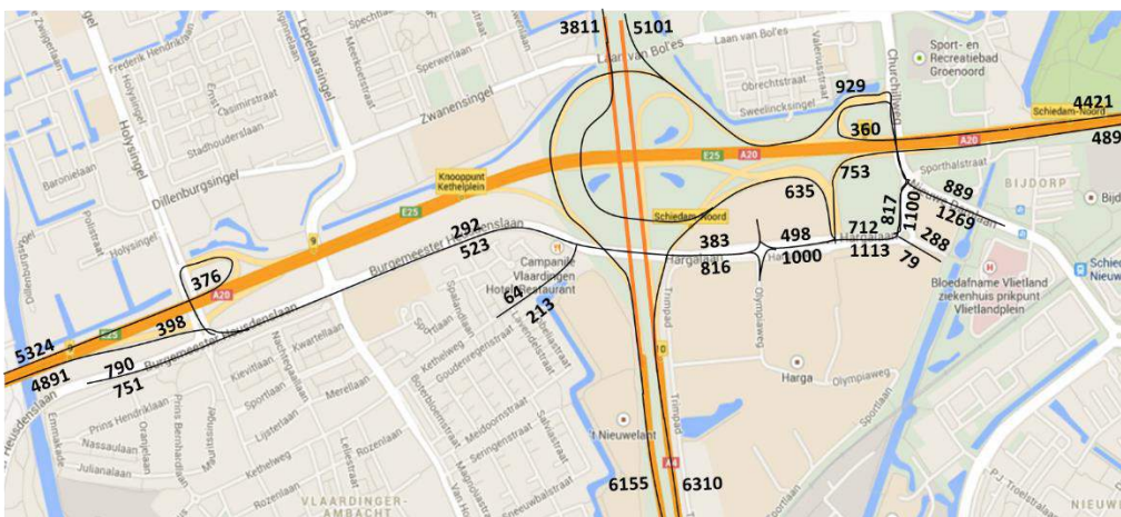
Figuur 4: Verkeersstromen ochtendspits 2020 bij ontwikkeling Decathlon en woonwijk [Bron: Google Maps]
