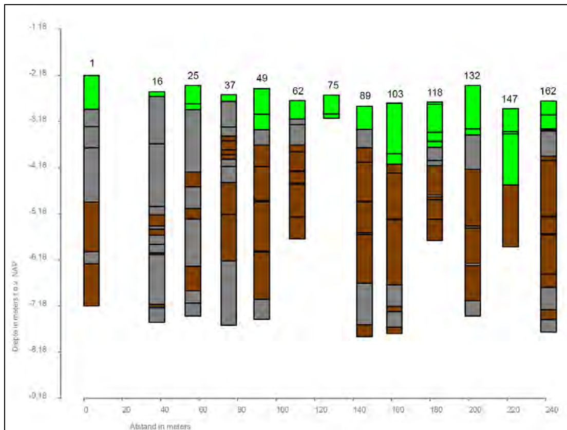
Afbeelding 22. Grafische weergave van de westelijke, diep doorgezette zuid-noord georiënteerde boorraai.
