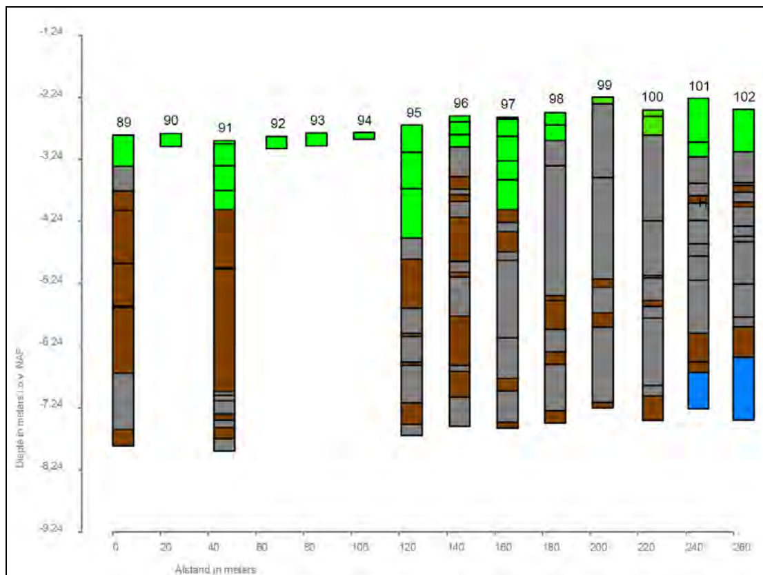
Afbeelding 15. Grafische weergave van Boring nr. 89 tot en met 102.
