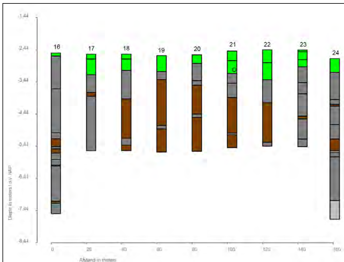
Afbeelding 9. Grafische weergave van Boring nr. 16 tot en met 24.
