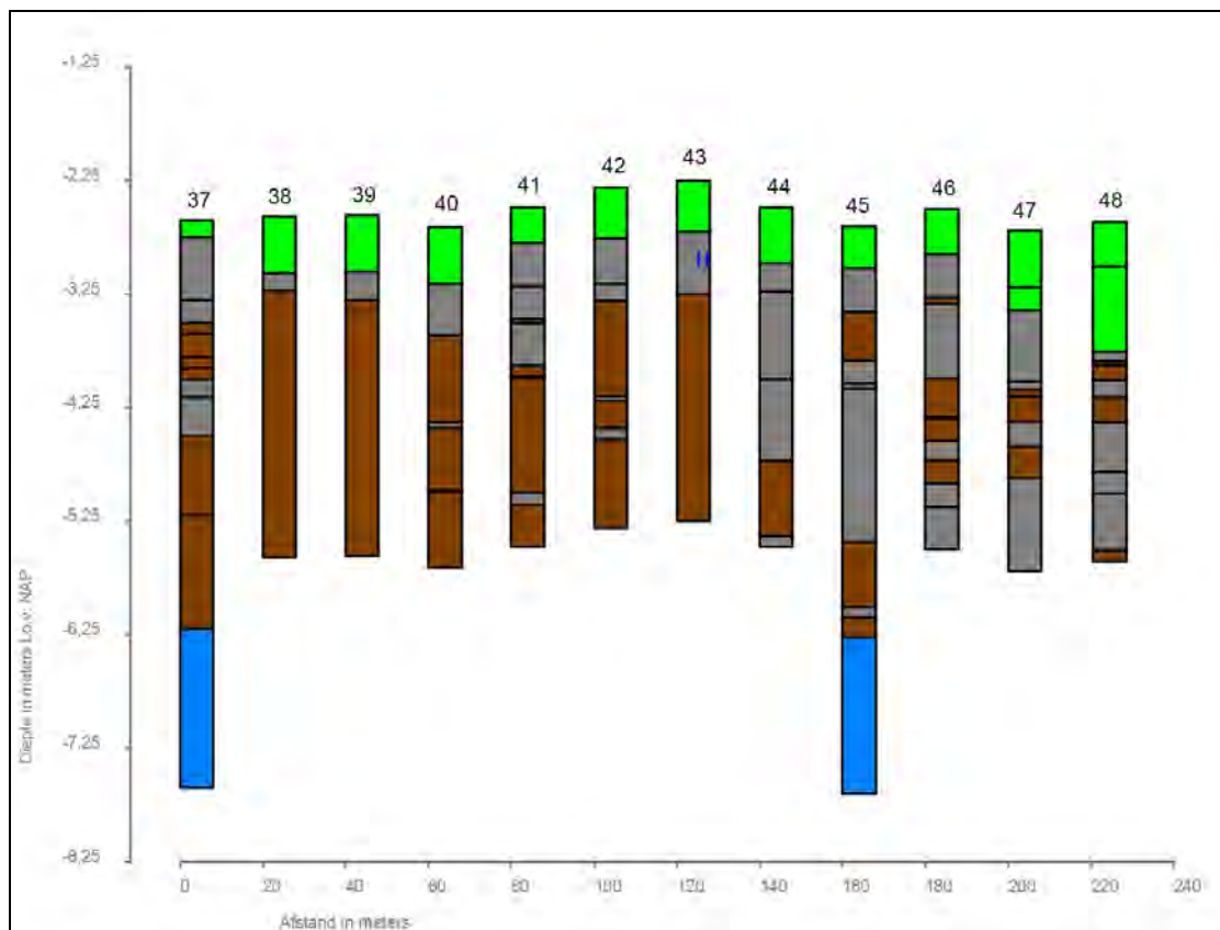
Afbeelding 11. Grafische weergave van Boring nr. 37 tot en met 48.
