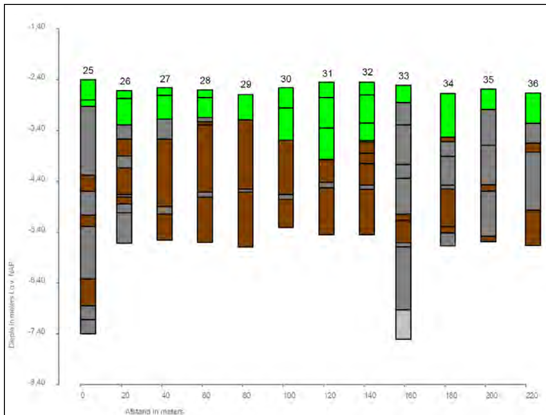
Afbeelding 10. Grafische weergave van Boring nr. 25 tot en met 36.
