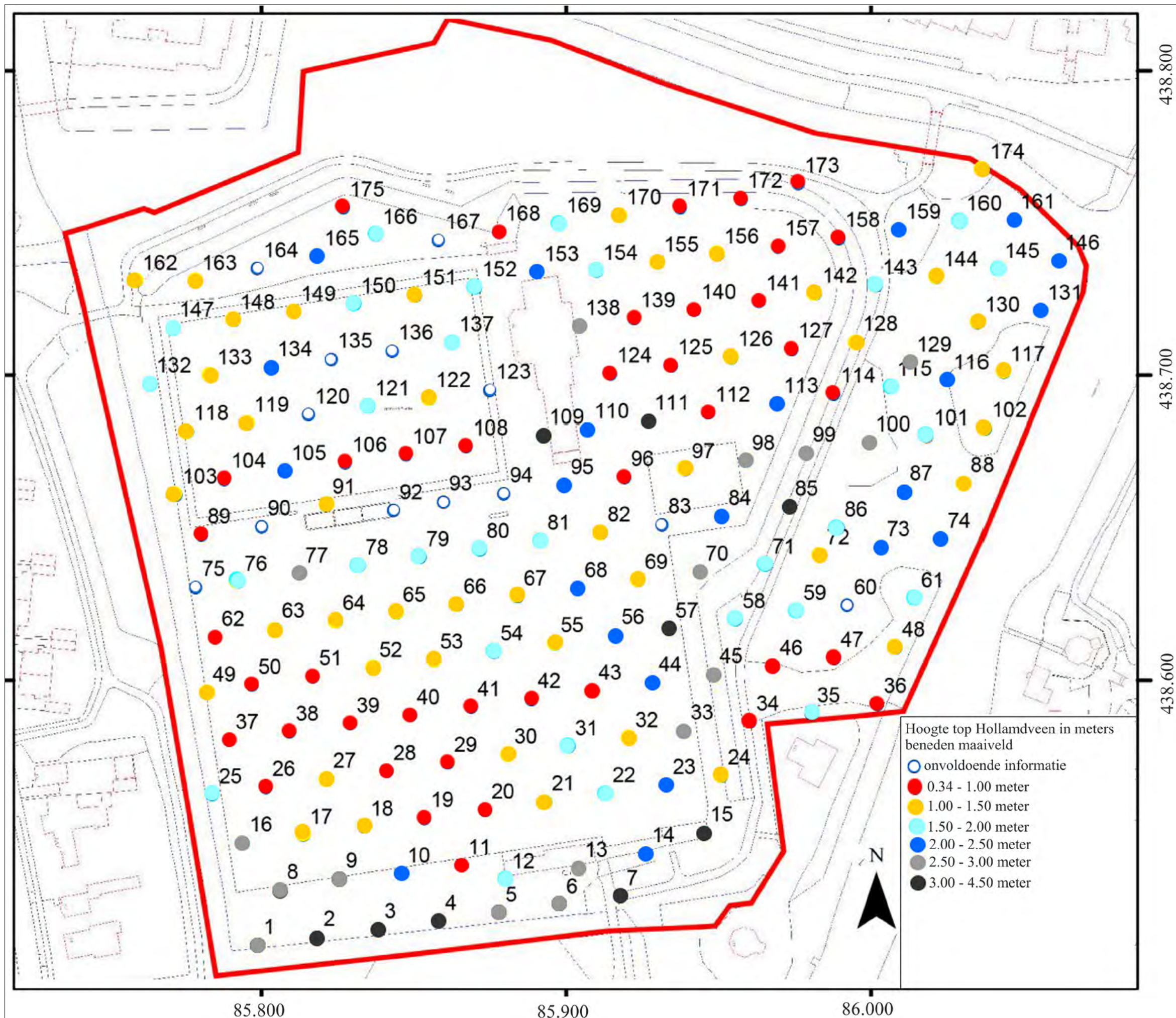
Afbeelding 27. De boorpuntenkaart van het IVO-Overig, met hoogte van de top van het Hollandveen in meters beneden het maaiveld.
