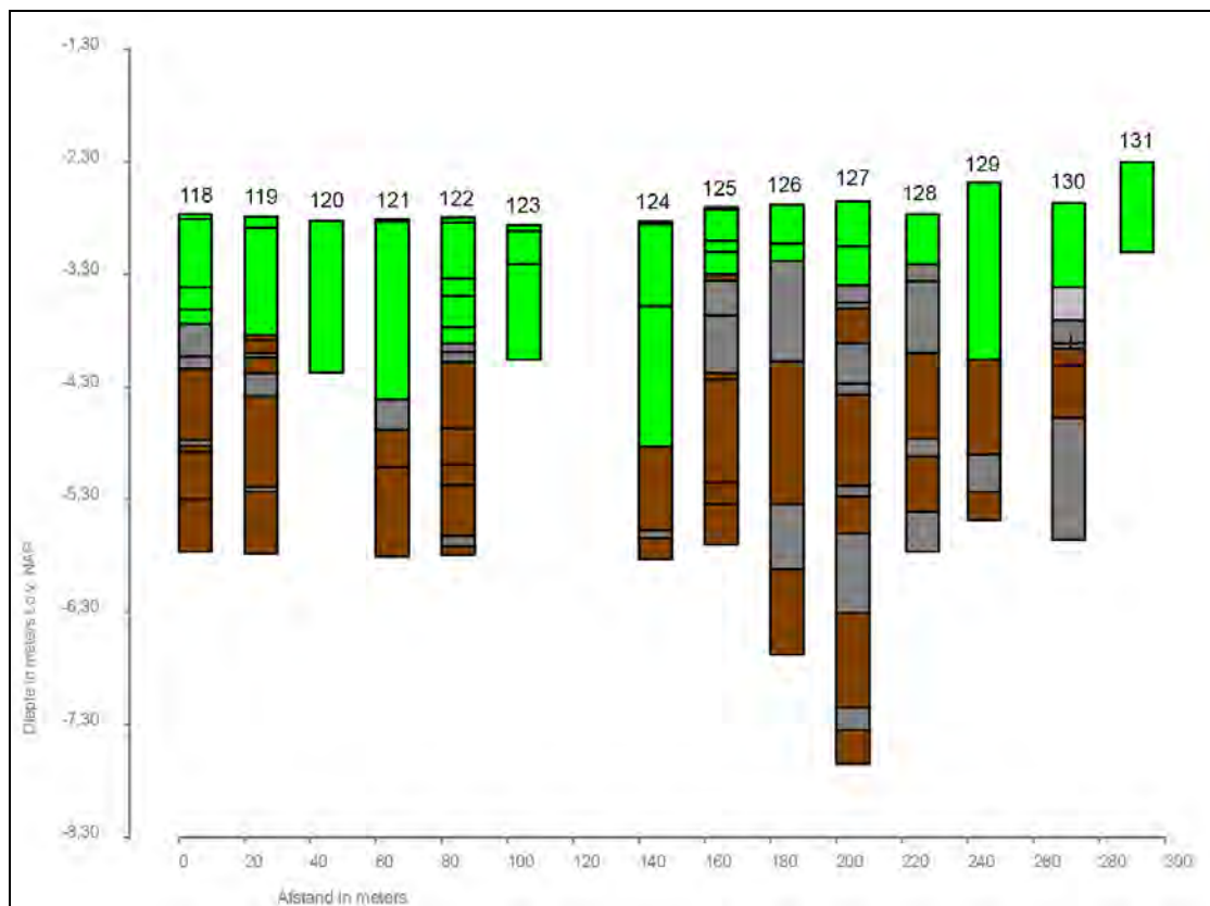
Afbeelding 17. Grafische weergave van Boring nr. 118 tot en met 131.
