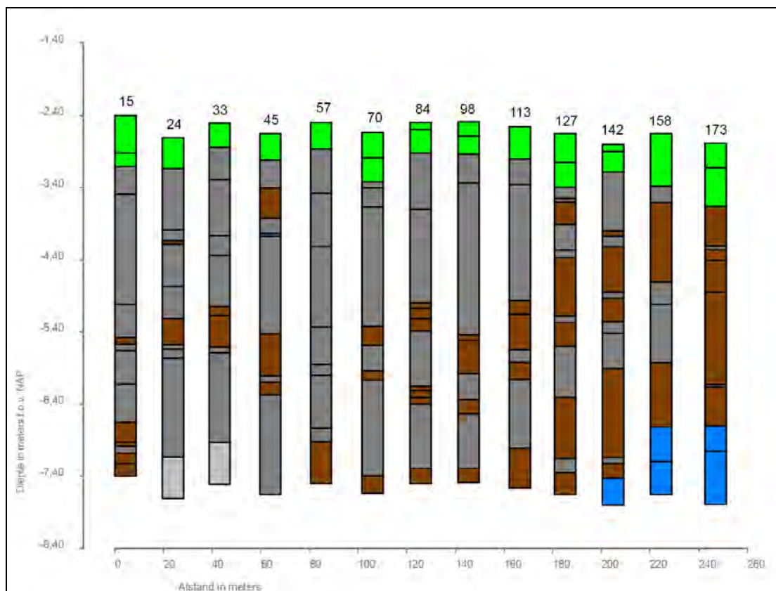
Afbeelding 23. Grafische weergave van de oostelijke, diep doorgezette zuid-noord georiënteerde boorraai.
