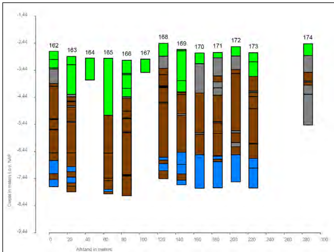
Afbeelding 20. Grafische weergave van Boring nr. 162 tot en met 174.
