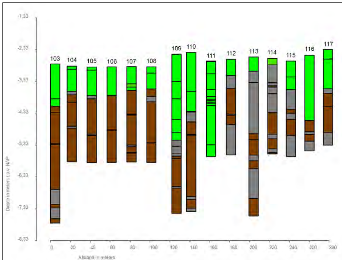
Afbeelding 16. Grafische weergave van Boring nr. 103 tot en met 117.
