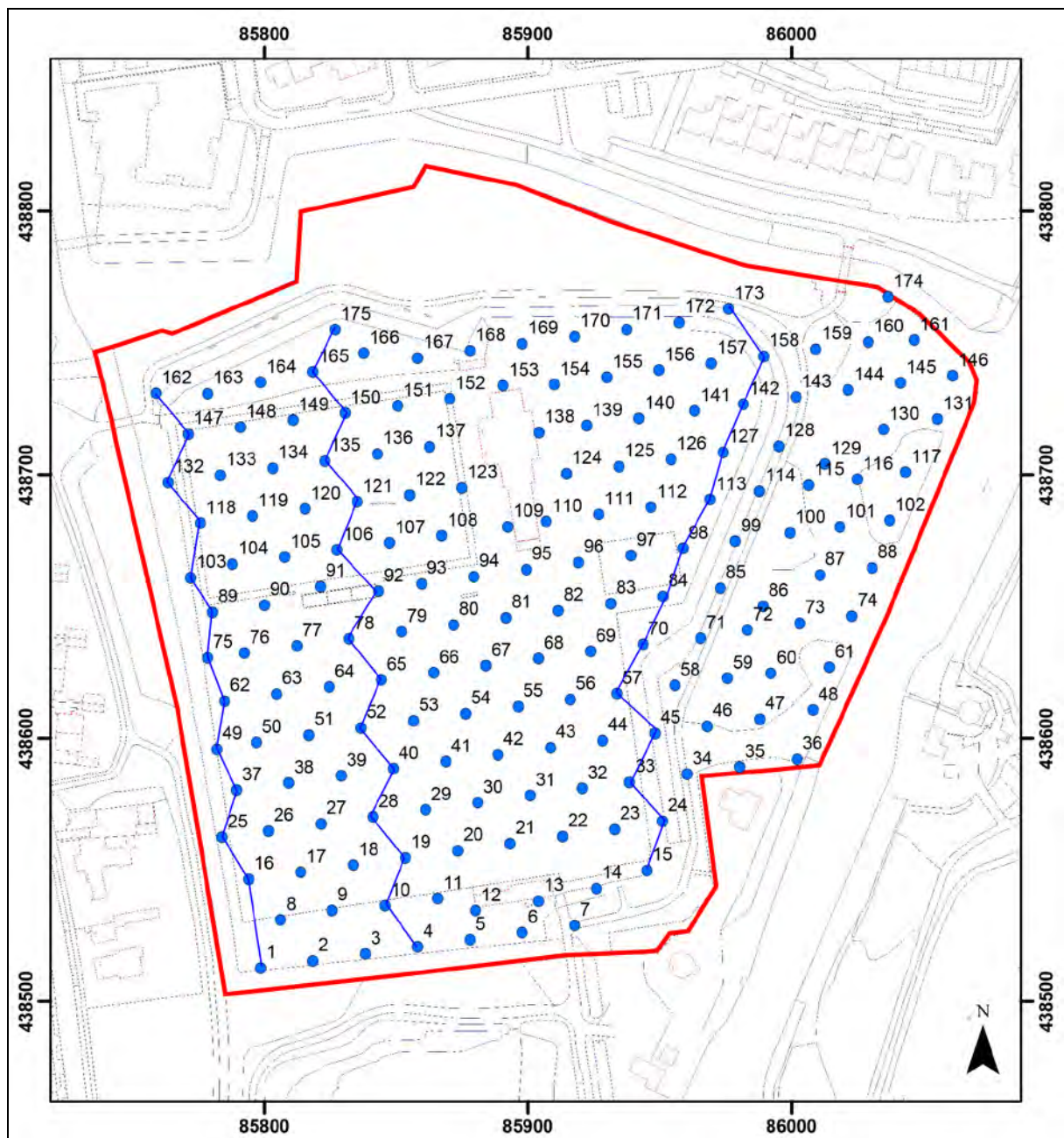
Afbeelding 6. De locaties van de boringen (in blauw), geprojecteerd op een uitsnede van de GBKN. Het plangebied is rood omkaderd. De locatie van de drie zuid-noordraaien zijn met een blauwe lijn gemarkeerd. De westelijke en de oostelijke raai zijn uitgevoerd tot op een diepte van 5 meter beneden het maaiveld. Bron GBKN: Topografische Dienst Kadaster, Emmen [2014]. Schaal 1: 2.500.
