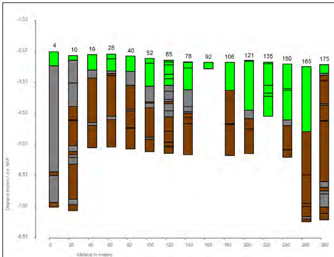
Afbeelding 24. Grafische weergave van de centraal gezette zuid-noord georiënteerde boorraai.
