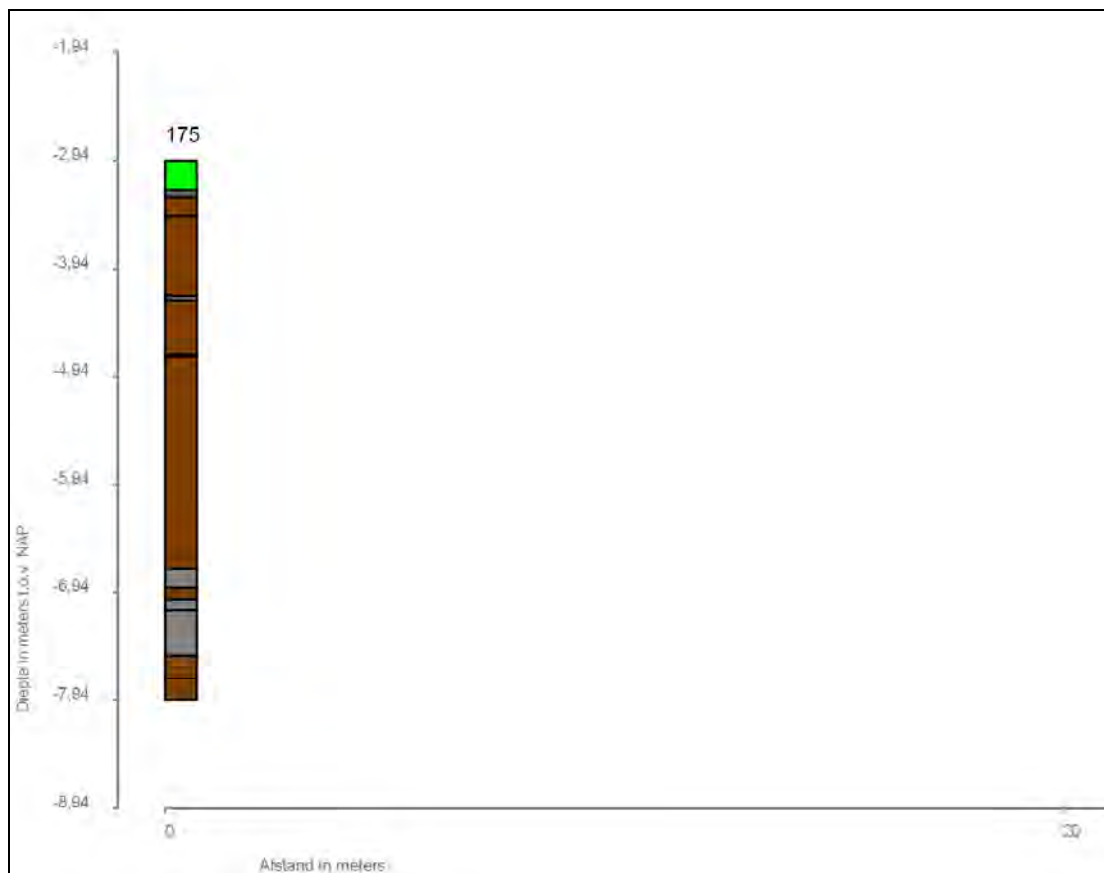
Afbeelding 21. Grafische weergave van Boring nr. 175.
