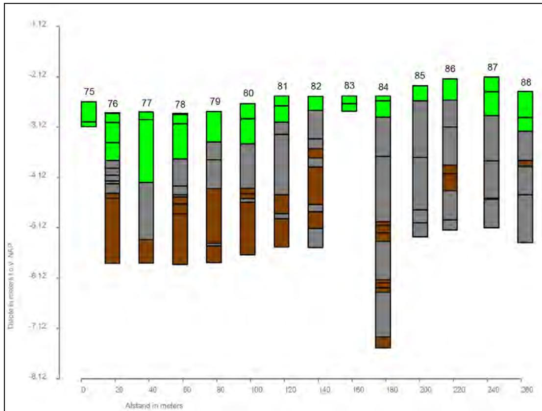
Afbeelding 14. Grafische weergave van Boring nr. 75 tot en met 88.
