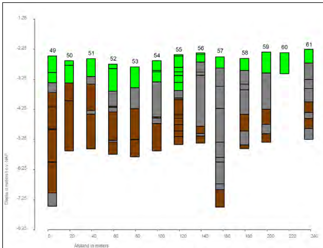
Afbeelding 12. Grafische weergave van Boring nr. 49 tot en met 61.
