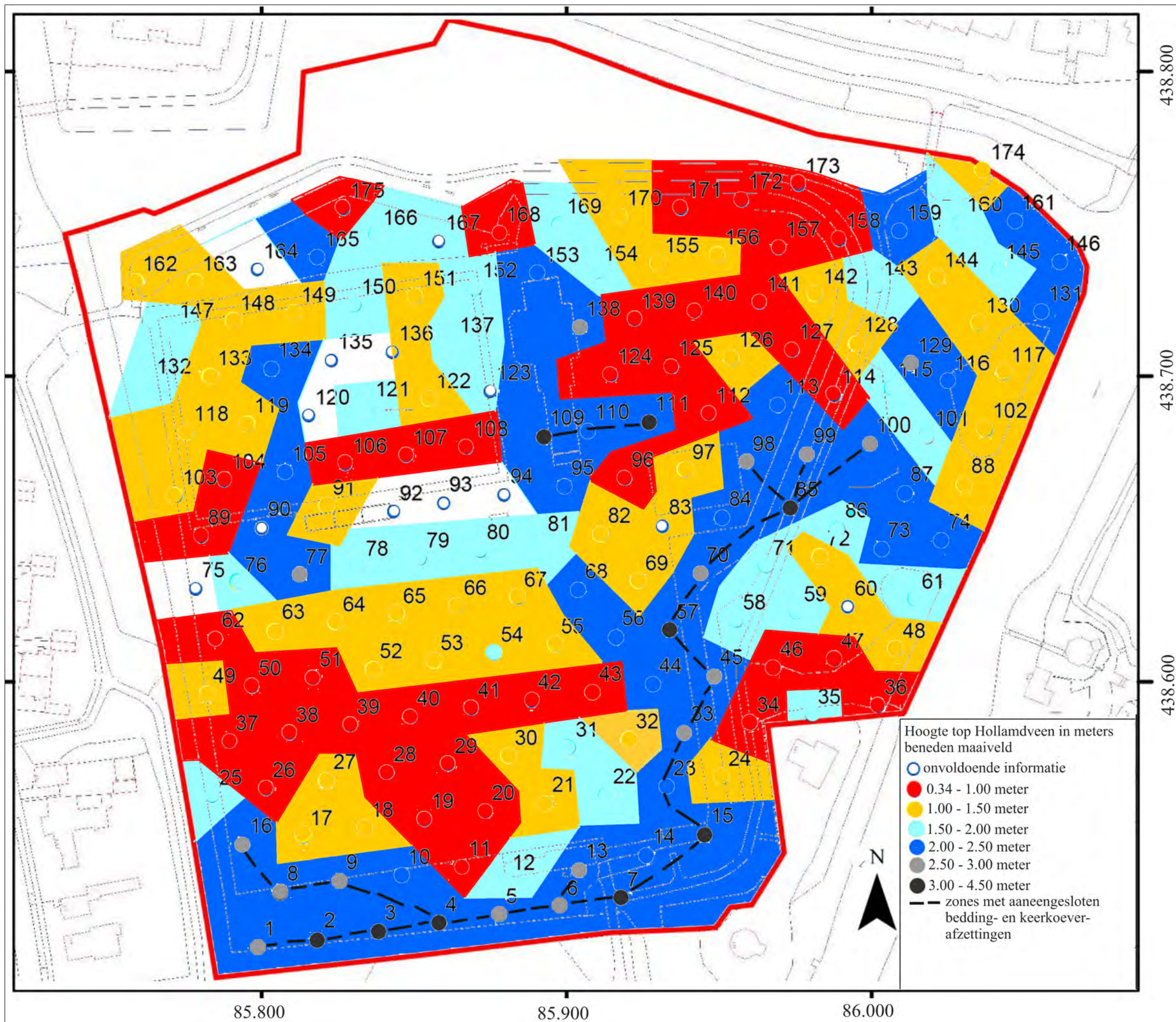
Afbeelding 28. De globale, schematische zonering van hoogte van de top van het Hollandveen, in meters beneden het maaiveld. Schaal 1: 1.250.
