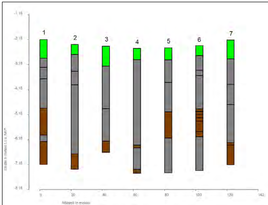
Afbeelding 7. Grafische weergave van Boring nr. 1 tot en met 7.
