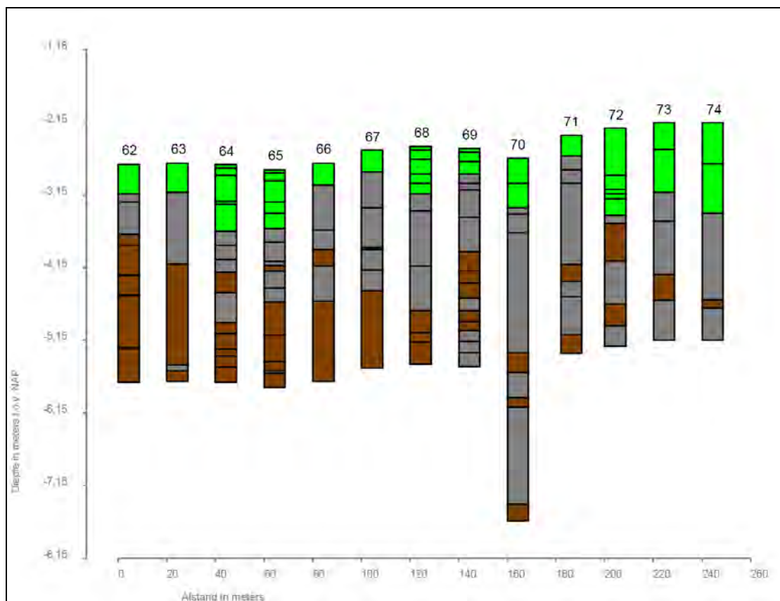
Afbeelding 13. Grafische weergave van Boring nr. 62 tot en met 74.
