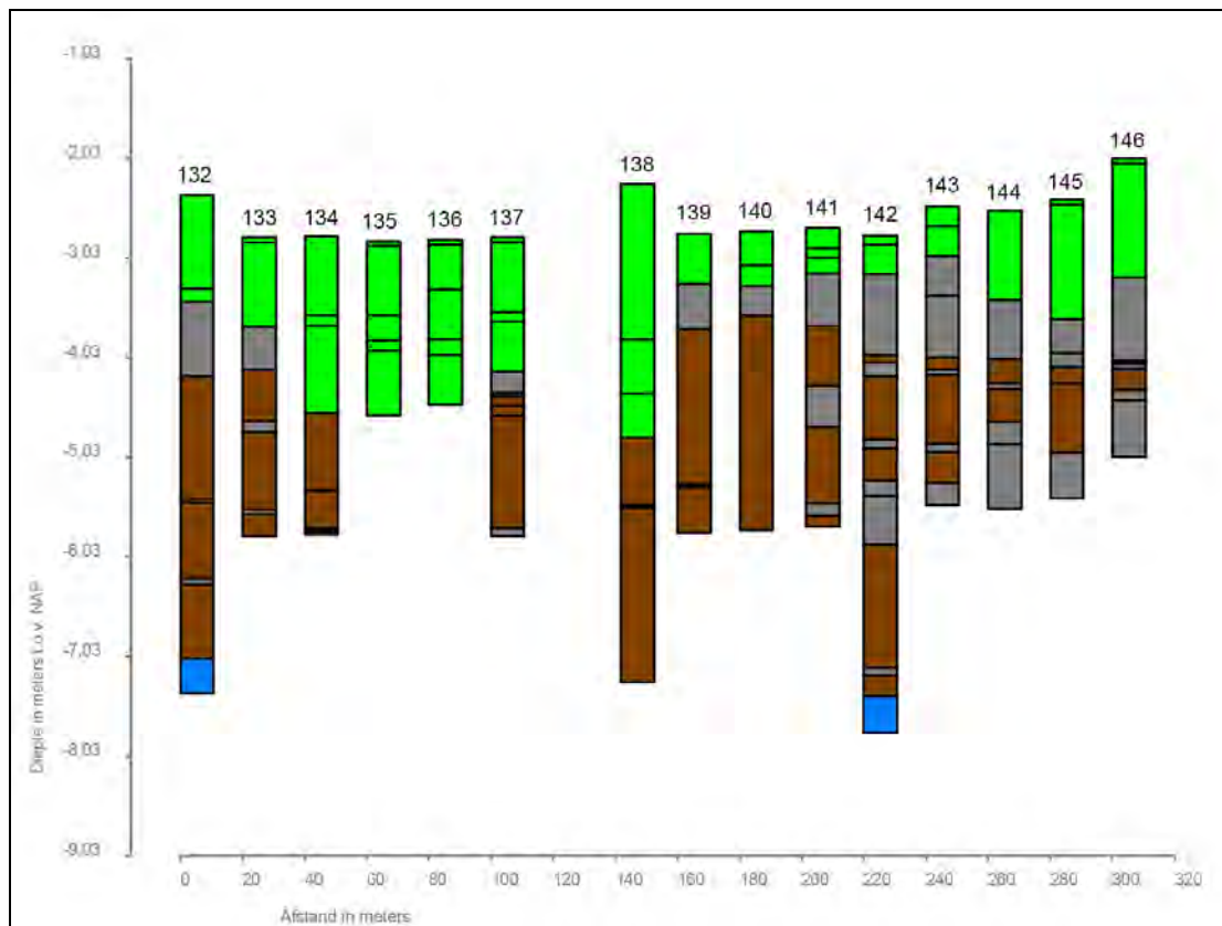
Afbeelding 18. Grafische weergave van Boring nr. 132 tot en met 146.
