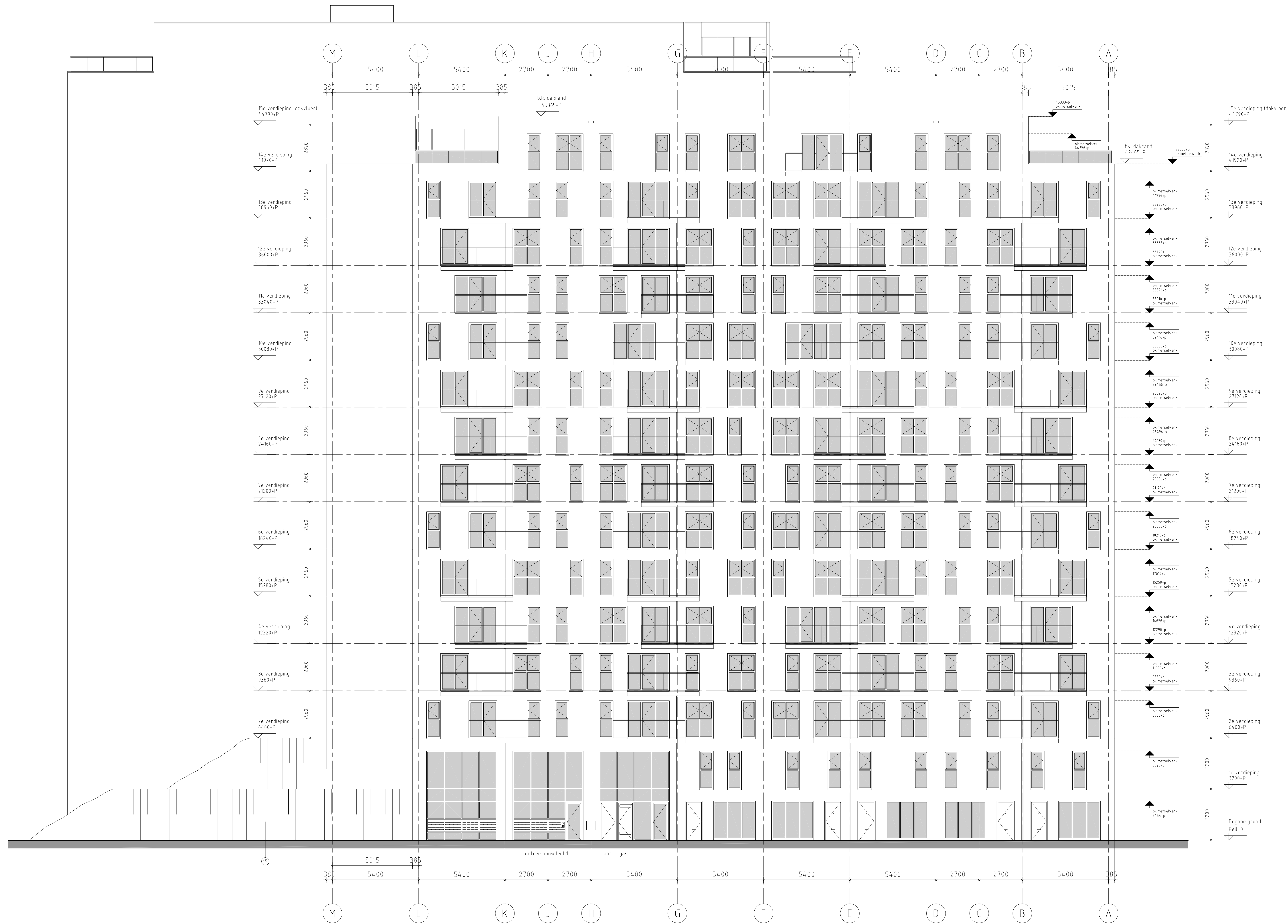
Westgevel bouwdeel 1
