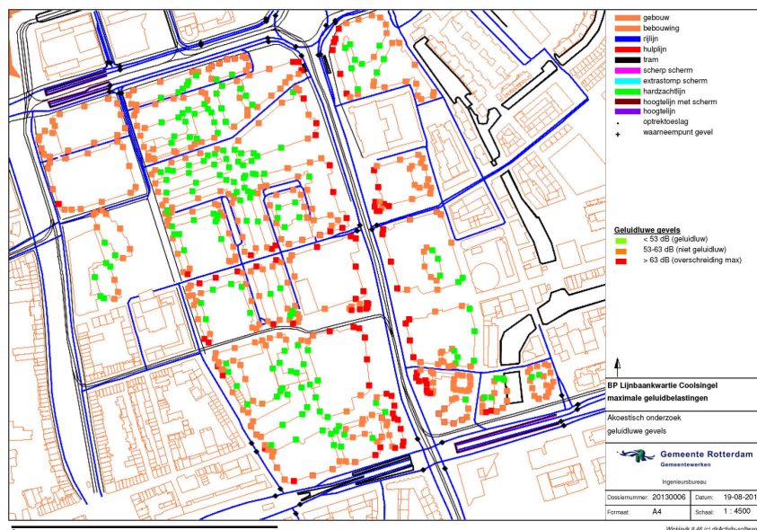
Figuur 5.1: Geluidluwe gevels voor wegverkeerslawaai
