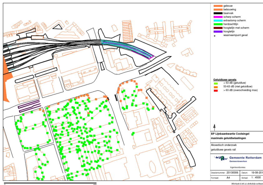
Figuur 5.2: Geluidluwe gevels voor railverkeerslawaaai
