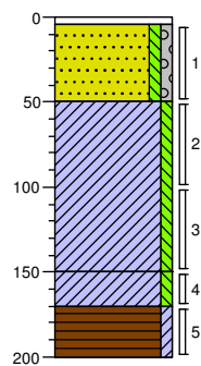
Boring/gat: 01
