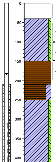
Boring/gat: 08
