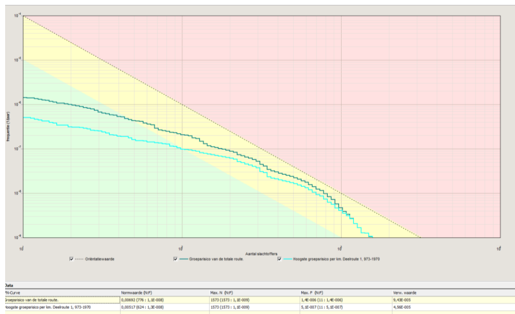
Grafiek 4.1: fN-curve berekend groepsrisico - huidige situatie
