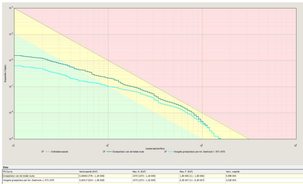
Grafiek 4.2: fN-curve berekend groepsrisico - toekomstige situatie
