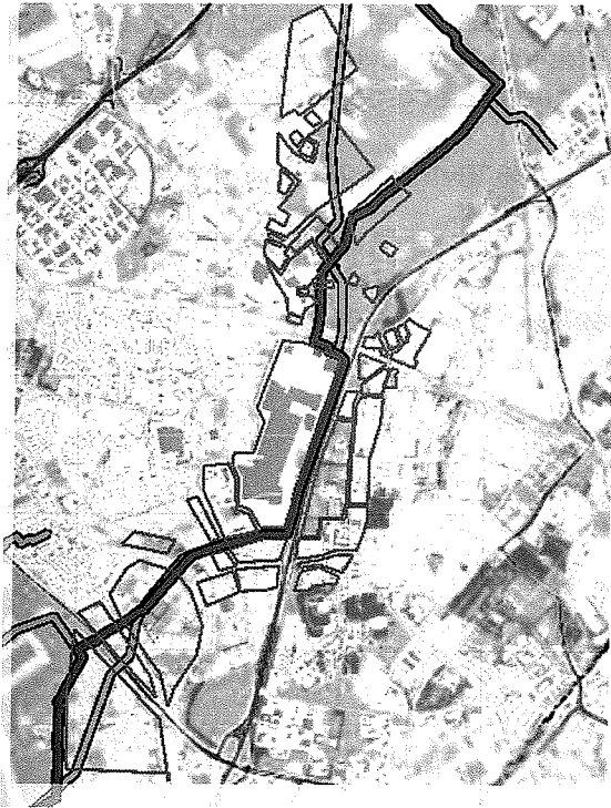
Figuur 8: — Kilometer leiding behorende bij de maximale overschrijding van de FN-curve voor W 535-01, — hoge druk aardgasleiding W535-01, — overige hoge druk aardgasleidingen.
