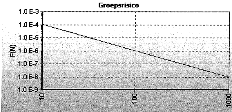
Figuur 16 Groepsrisicodiagram (of FN curve) voor W535-01, — groepsrisico curve, — oriëntatiewaarde
