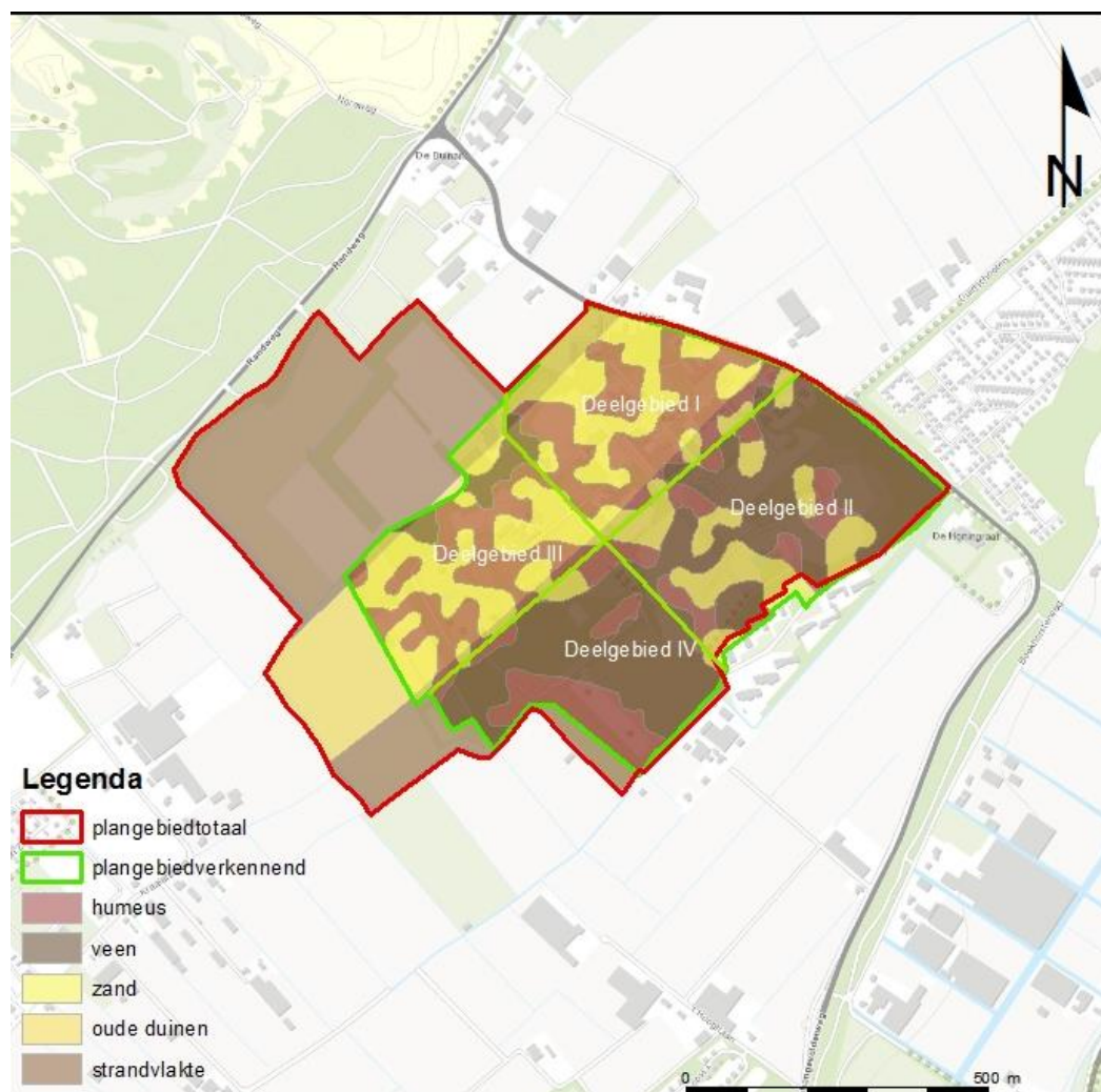
Figuur 4 reconstructie van het landschap en de sedimenten op basis van de boringen van Wilgen (2003). De code humeus betekent dat er in de boringen één of meerdere humeuze zandlagen voorkomen in het zandpakket. Bij de code zand komt in de boring alleen een pakket bruin of grijs zand voor.
