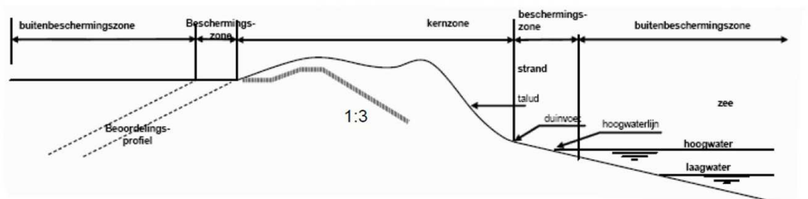
Afbeelding 12: boven: keurzones, onder: beoordelingsprofiel hybride constructie "dijk in duin (afbeeldingen afkomstig uit Deel II 'Beleidsregels' van de Kustnota)
