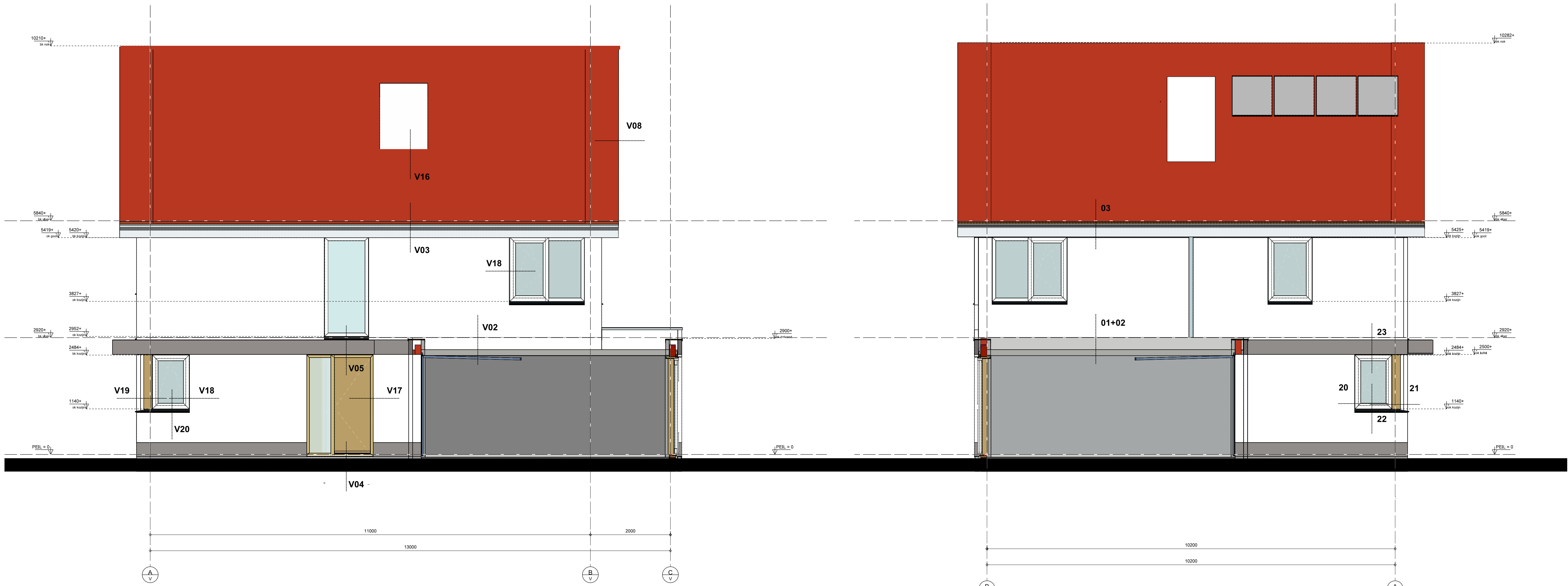
RECHTERZIJGEVEL
