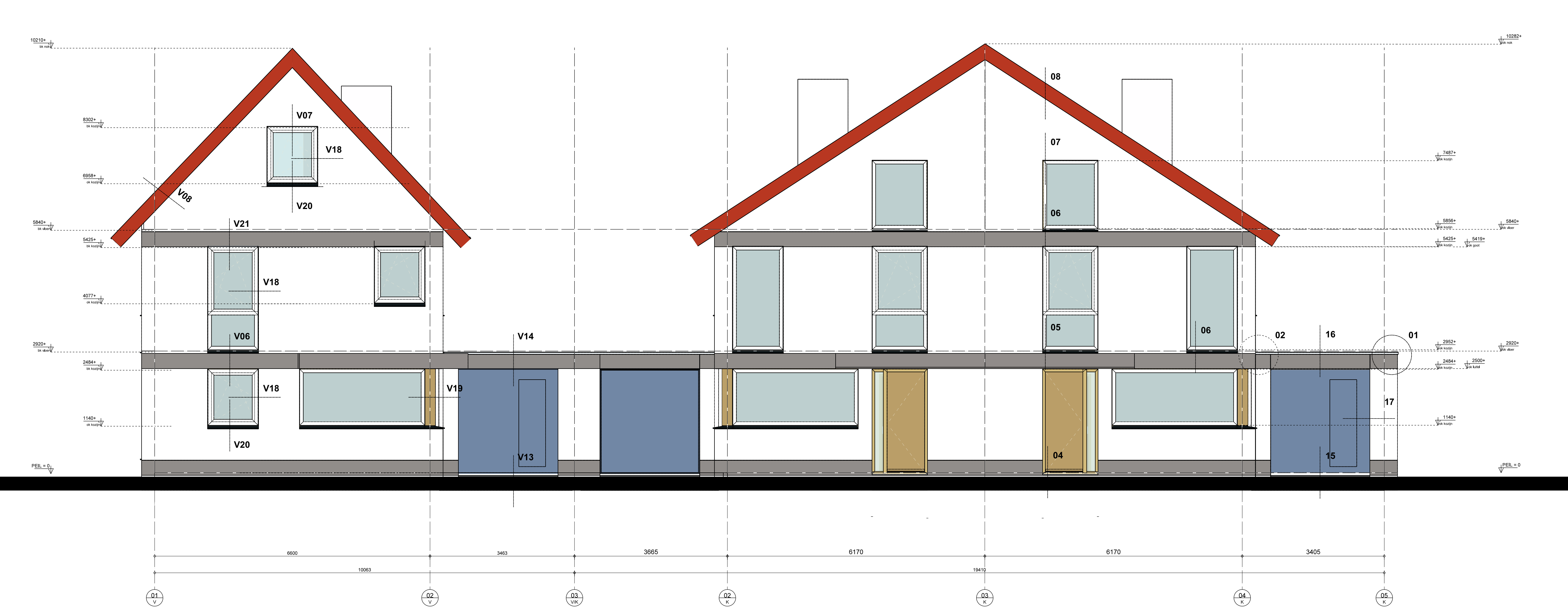
VOERGEVEL
