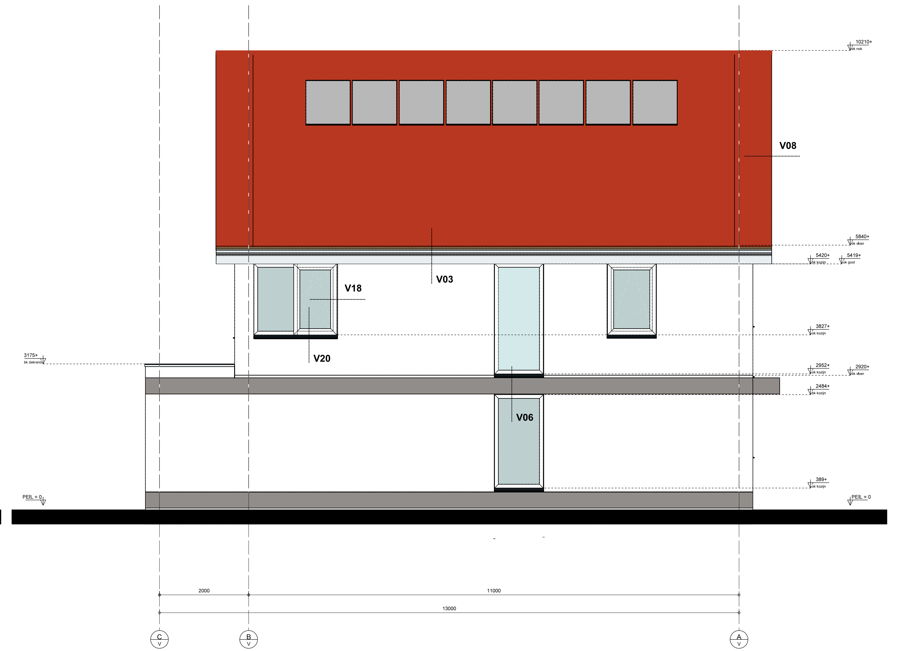
LINKERZIJGEVEL
