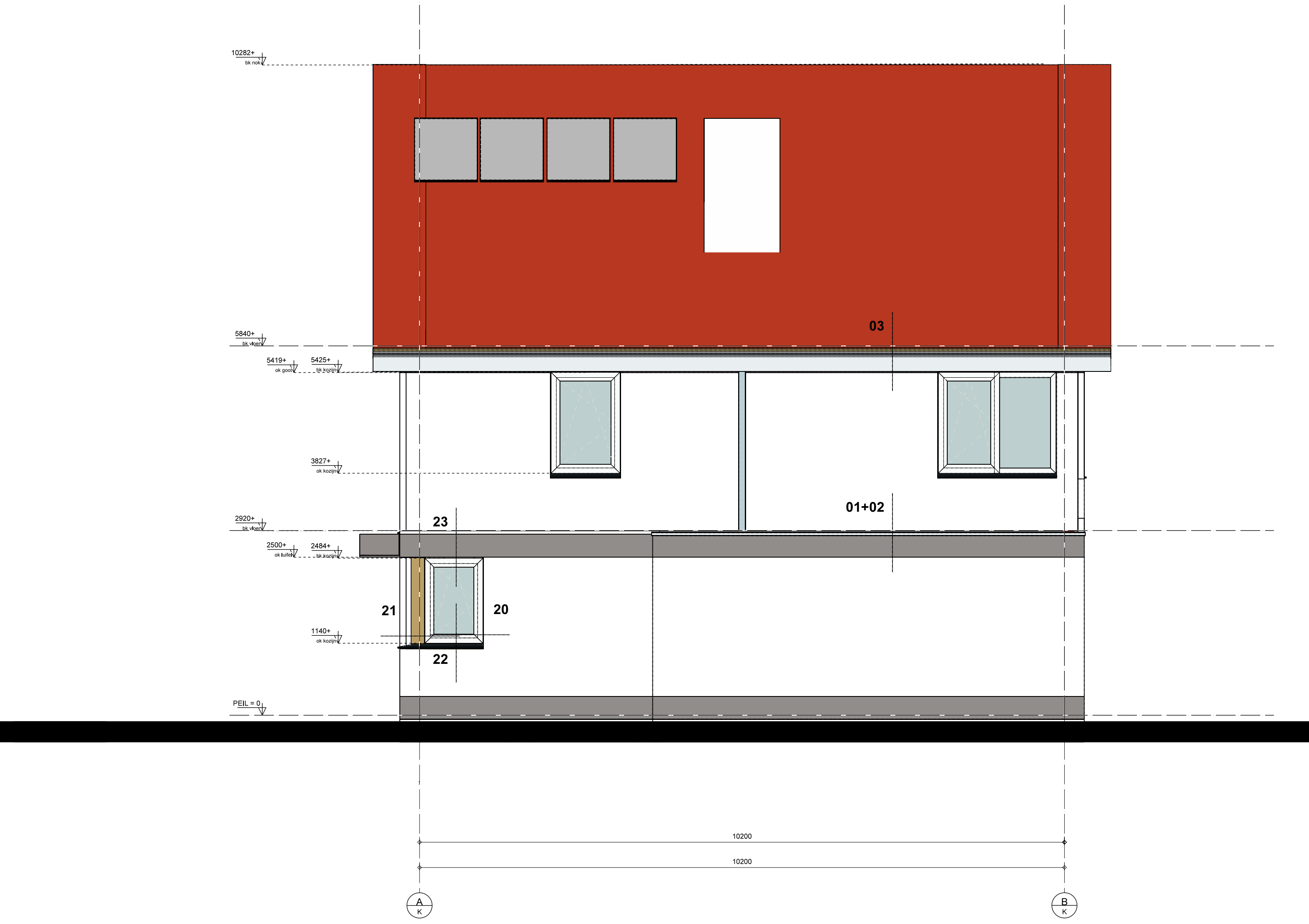
RECHTERZIJGEVEL
