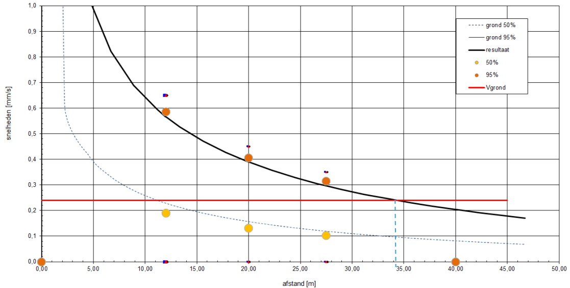
Figuur 4.1: Fit van trillingsintensiteit treinpassages (95%-waarden) - afstand (m) versus trillingsnelheid (mms/)
