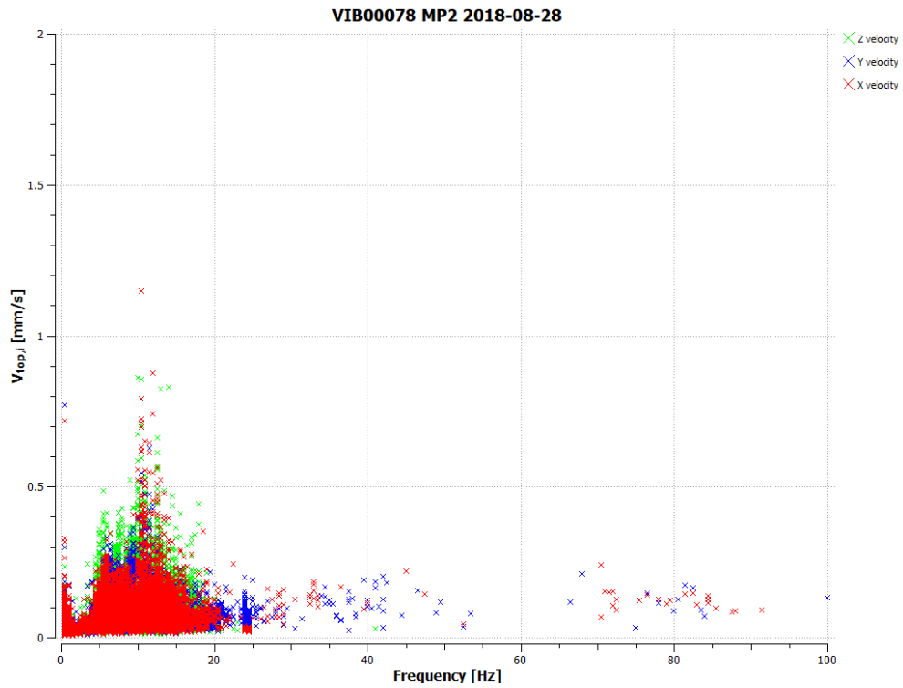
Figuur 3.5: Frequentie-Snelheid MP2
