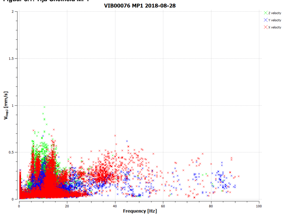
Figuur 3.2: Frequentie-Snelheid MP1
