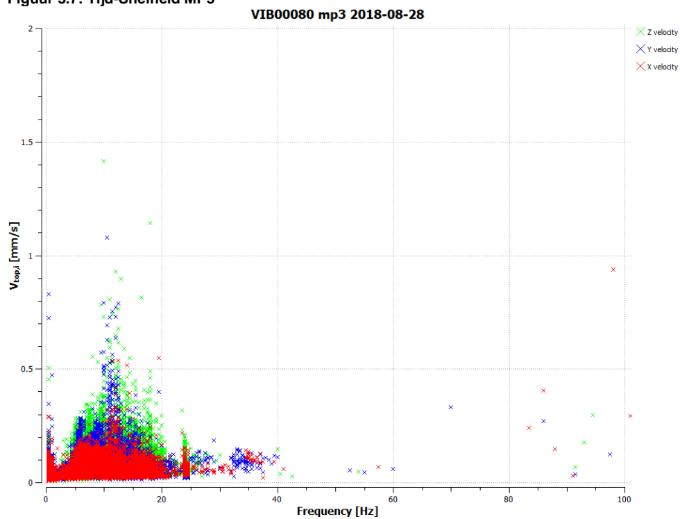
Figuur 3.8: Frequentie-Snelheid MP3
