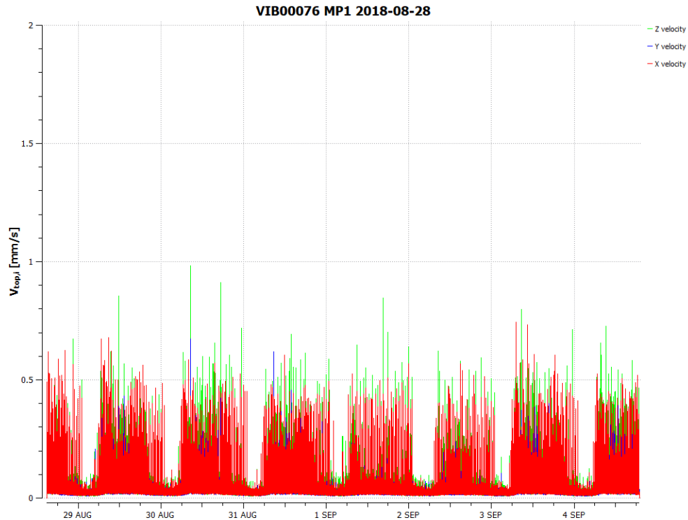
Figuur 3.1: Tijd-Snelheid MP1
