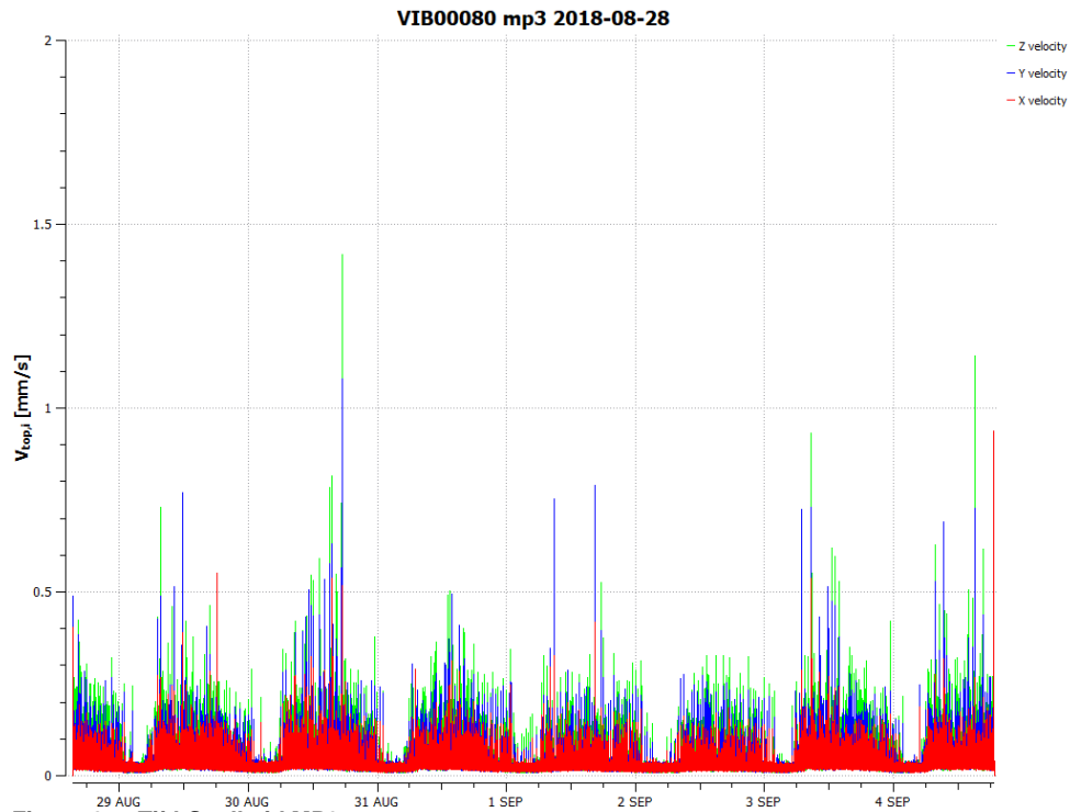
Figuur 3.7: Tijd-Snelheid MP3
