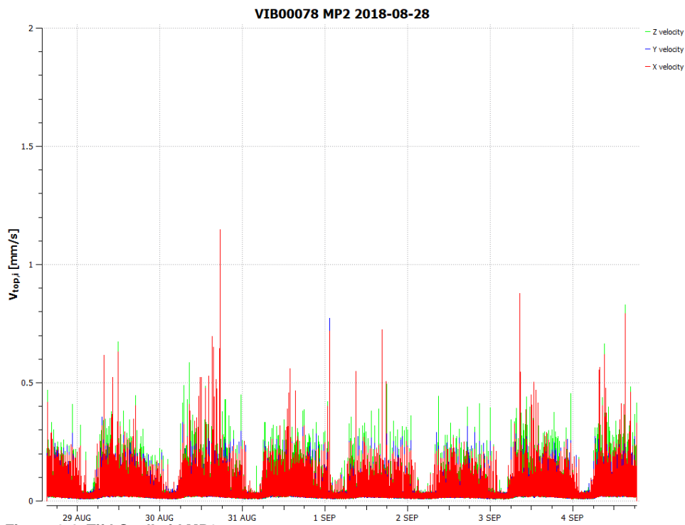
Figuur 3.4: Tijd-Snelheid MP2
