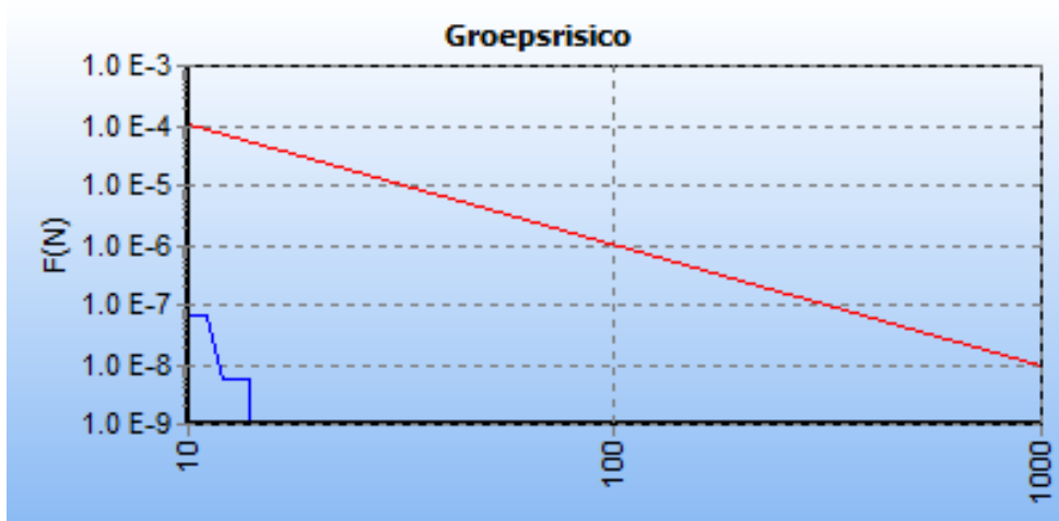
Figuur 5.3 FN curve voor W-513-02 van N.V. Nederlandse Gasunie voor de kilometer tussen stationing 1020.00 en stationing 2020.00
