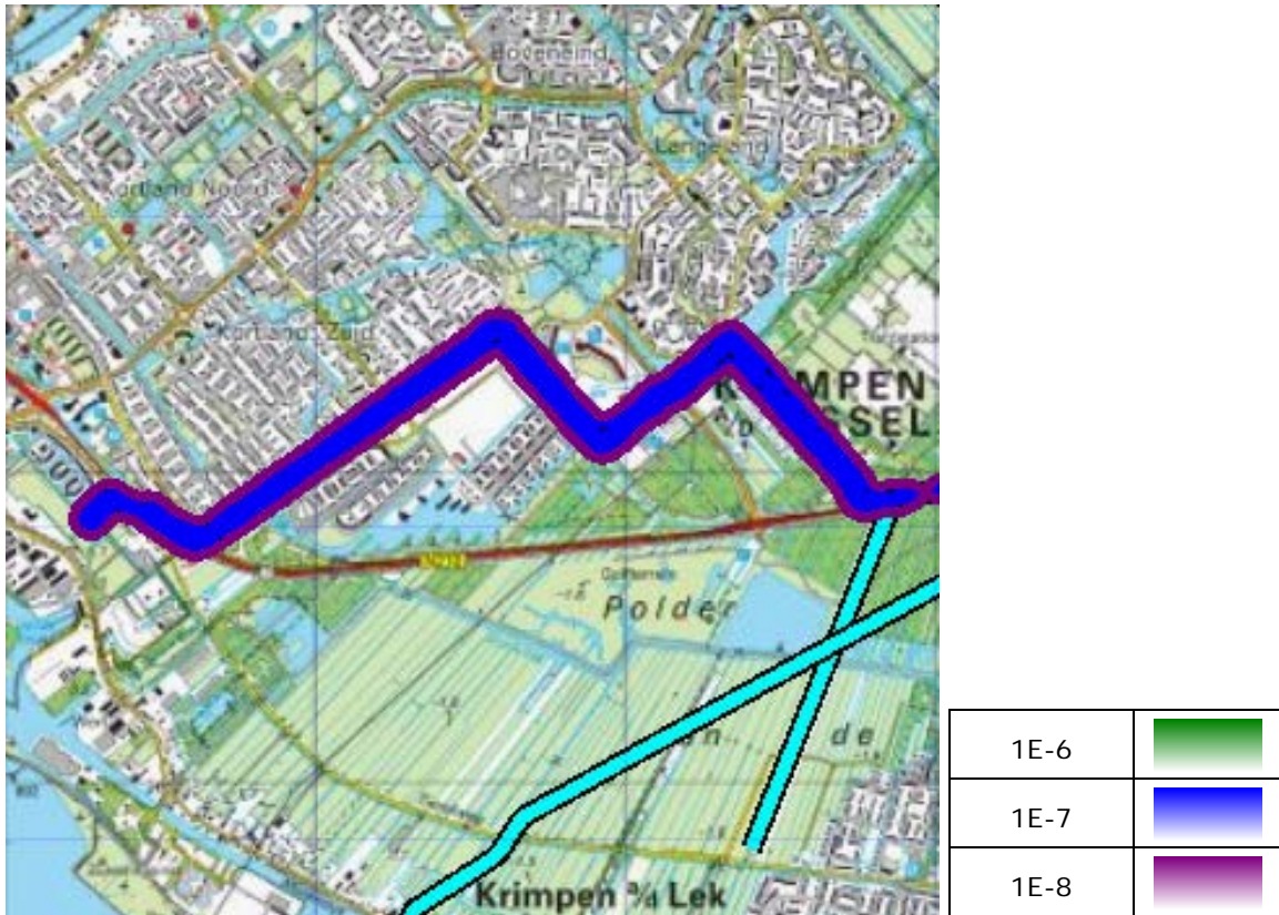
Figuur 4.1 Plaatsgebonden risico voor W-513-02 van N.V. Nederlandse Gasunie
