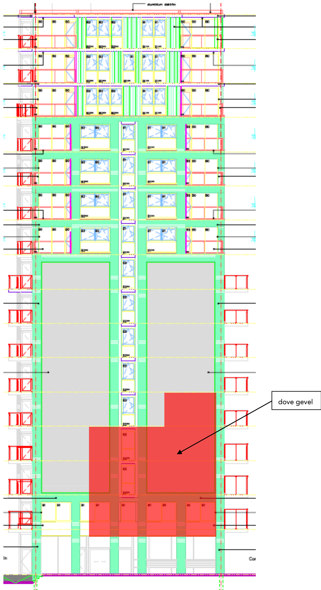
Figuur 10 – overzicht dove gevels
