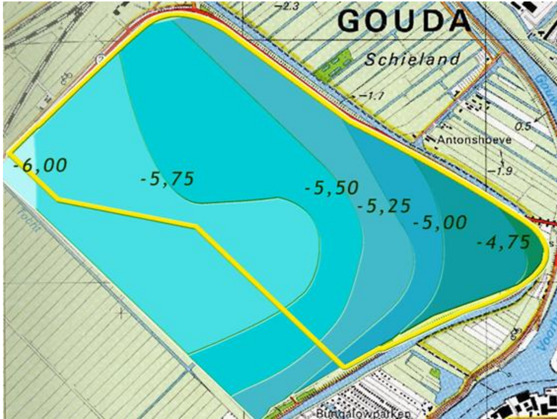
Afbeelding 4.4 Grondwaterstanden Westergouwe (bron: Projectbureau Westergouwe)
