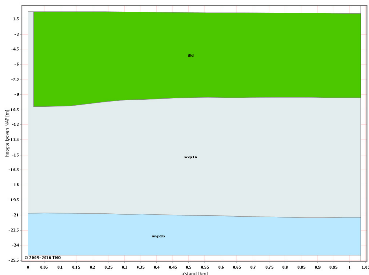
Figuur 2. Geohydrologisch model
