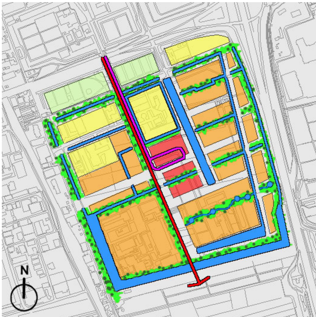
Afbeelding 2 stedenbouwkundige structuur
