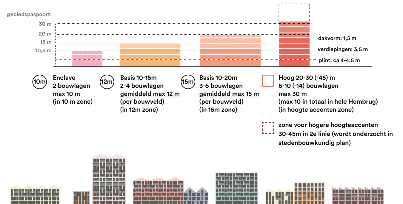
Masterplan: wisselende bouwhoogtes, genereuse verdiepingshoogtes en interessante dakvormen
