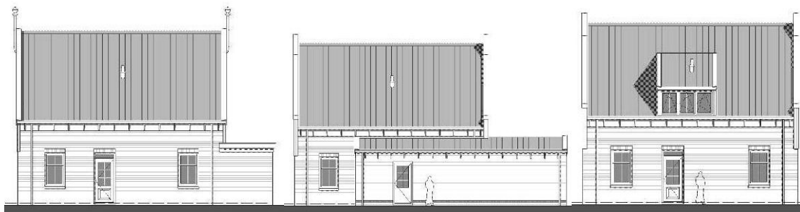
ZIJGEVEL - RECHTS
