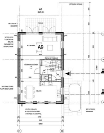
BEGANE GROND
