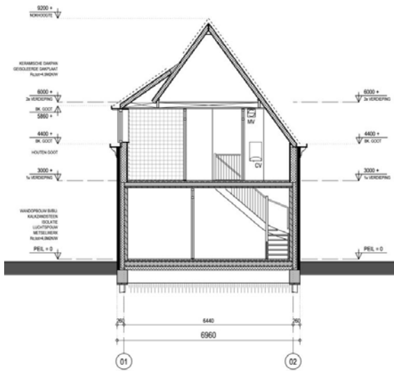
DOORSNEDE A
