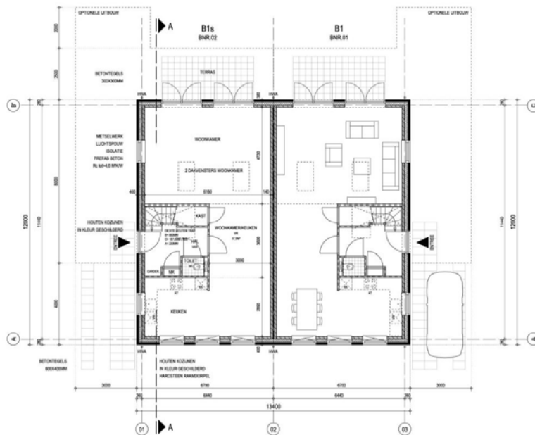
BEGANE GROND
