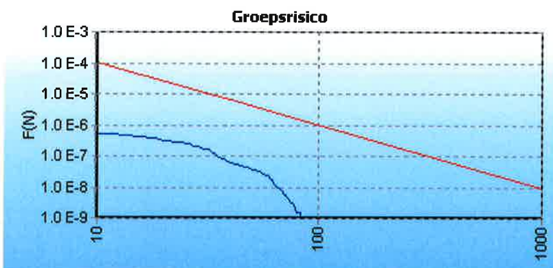
5.5 Figuur 5.5 FN curve voor W-532-01 van N.V. Nederlandse Gasunie voor de kilometer tussen stationing 7860.00 en stationing 8860.00
