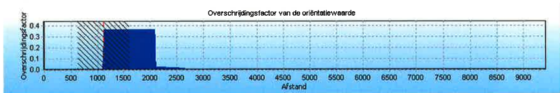
4.6 Figuur 4.6 Groepsrisico screening voor W-532-02 van N.V. Nederlandse Gasunie
