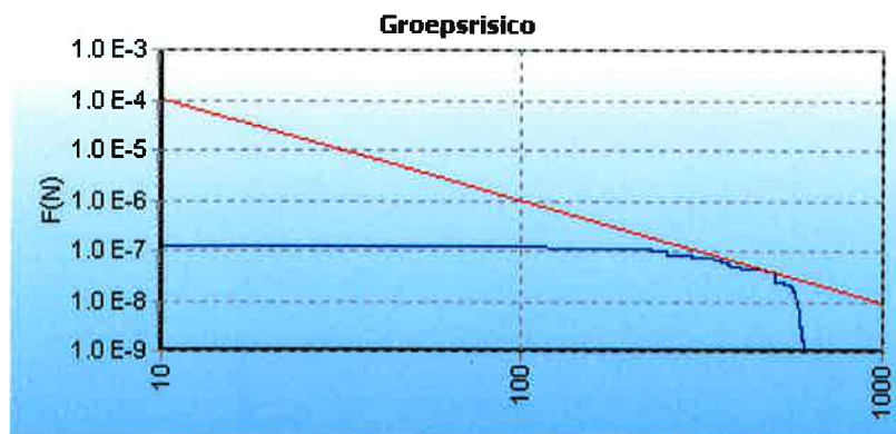
5.4 Figuur 5.4 FN curve voor A-611-01 van N.V. Nederlandse Gasunie voor de kilometer tussen stationing 0.00 en stationing 0.00
