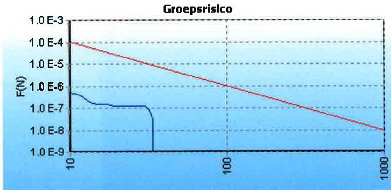
5.13 Figuur 5.13 FN curve voor W-534-09 van N.V. Nederlandse Gasunie voor de kilometer tussen stationing 0.00 en stationing 0.00
