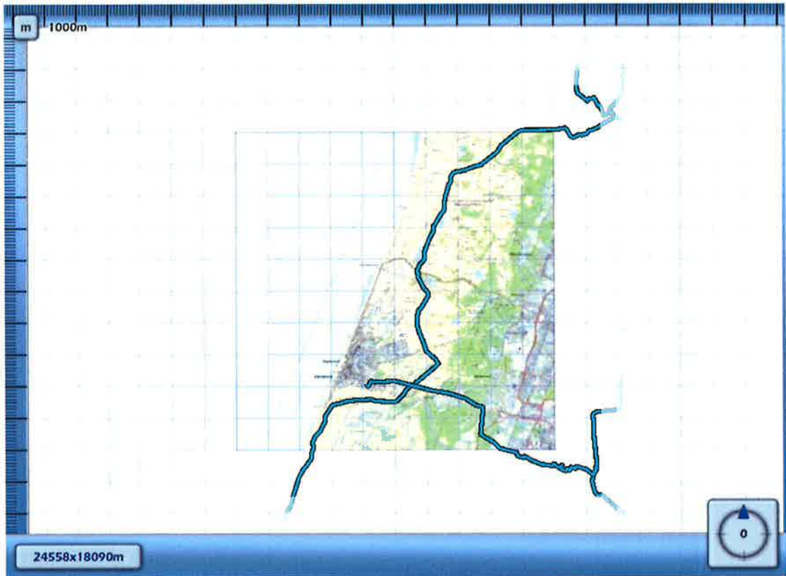
3.13 Figuur 3.13 Plaatsgebonden risico voor W-534-09 van N.V. Nederlandse Gasunie
