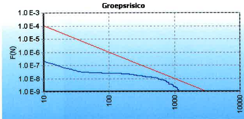
5.7 Figuur 5.7 FN curve voor W-532-03 van N.V. Nederlandse Gasunie voor de kilometer tussen stationing 0.00 en stationing 0.00
