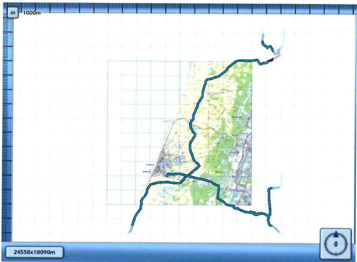
3.14 Figuur 3.14 Plaatsgebonden risico voor W-534-22 van N.V. Nederlandse Gasunie
