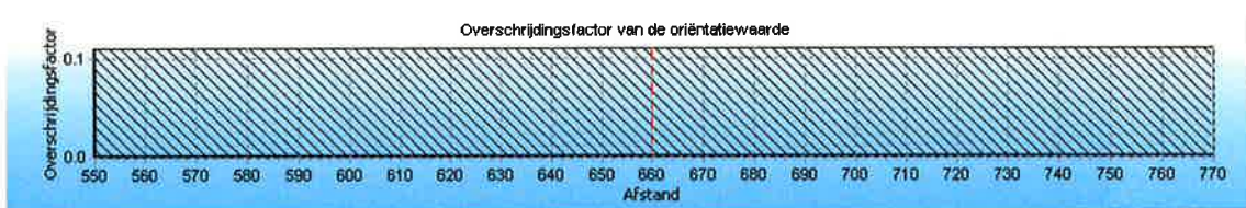
4.14 Figuur 4.14 Groepsrisico screening voor W-534-22 van N.V. Nederlandse Gasunie
