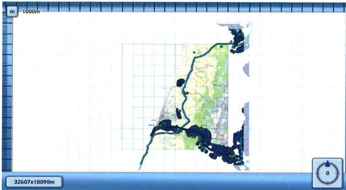
4.7 Figuur 4.7 Groepsrisico screening voor W-532-03 van N.V. Nederlandse Gasunie
