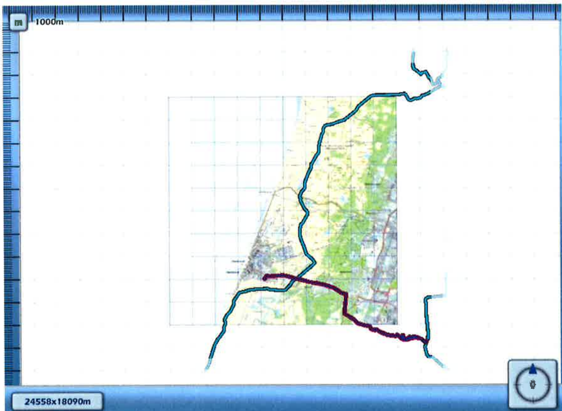
3.6 Figuur 3.6 Plaatsgebonden risico voor W-532-02 van N.V. Nederlandse Gasunie
