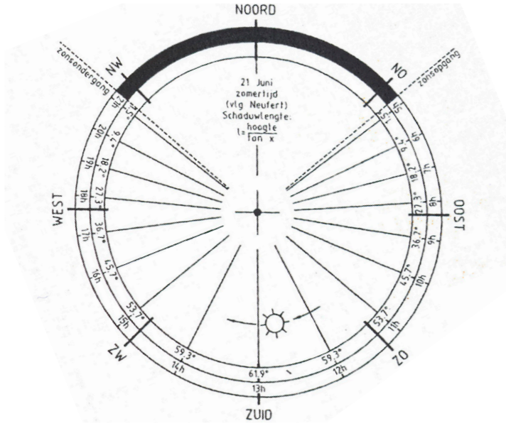
zonnediagram zomer
