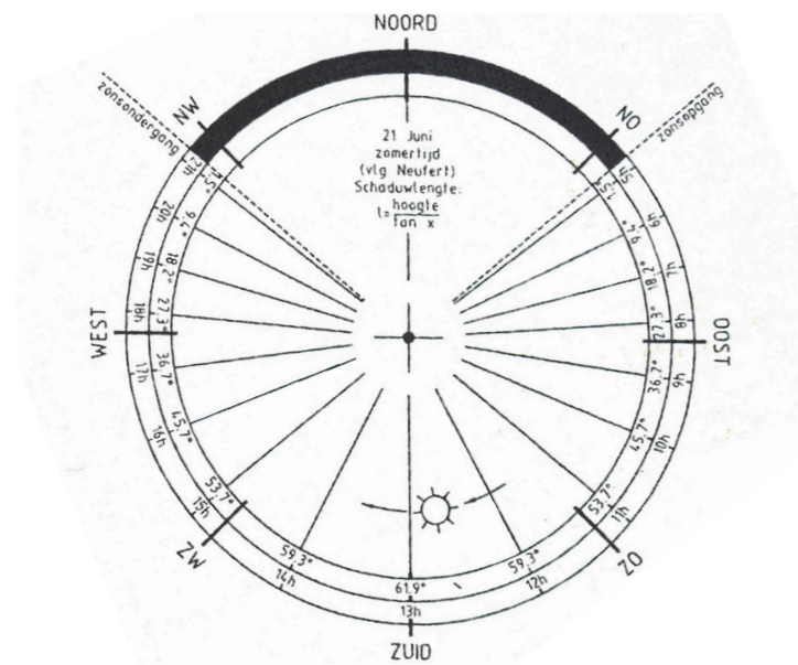
zonedigram zomer
