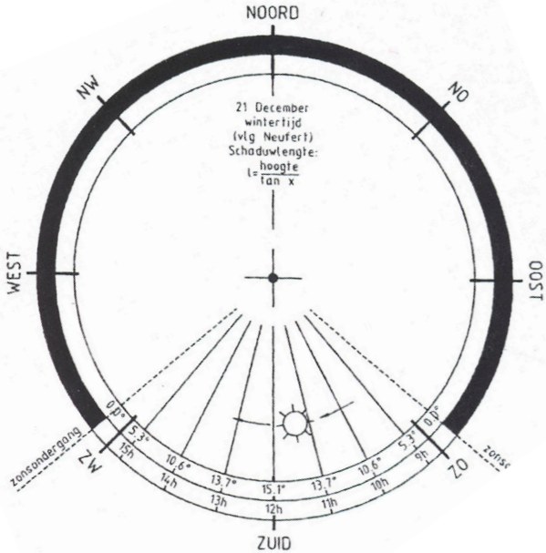
zonedigram winter
