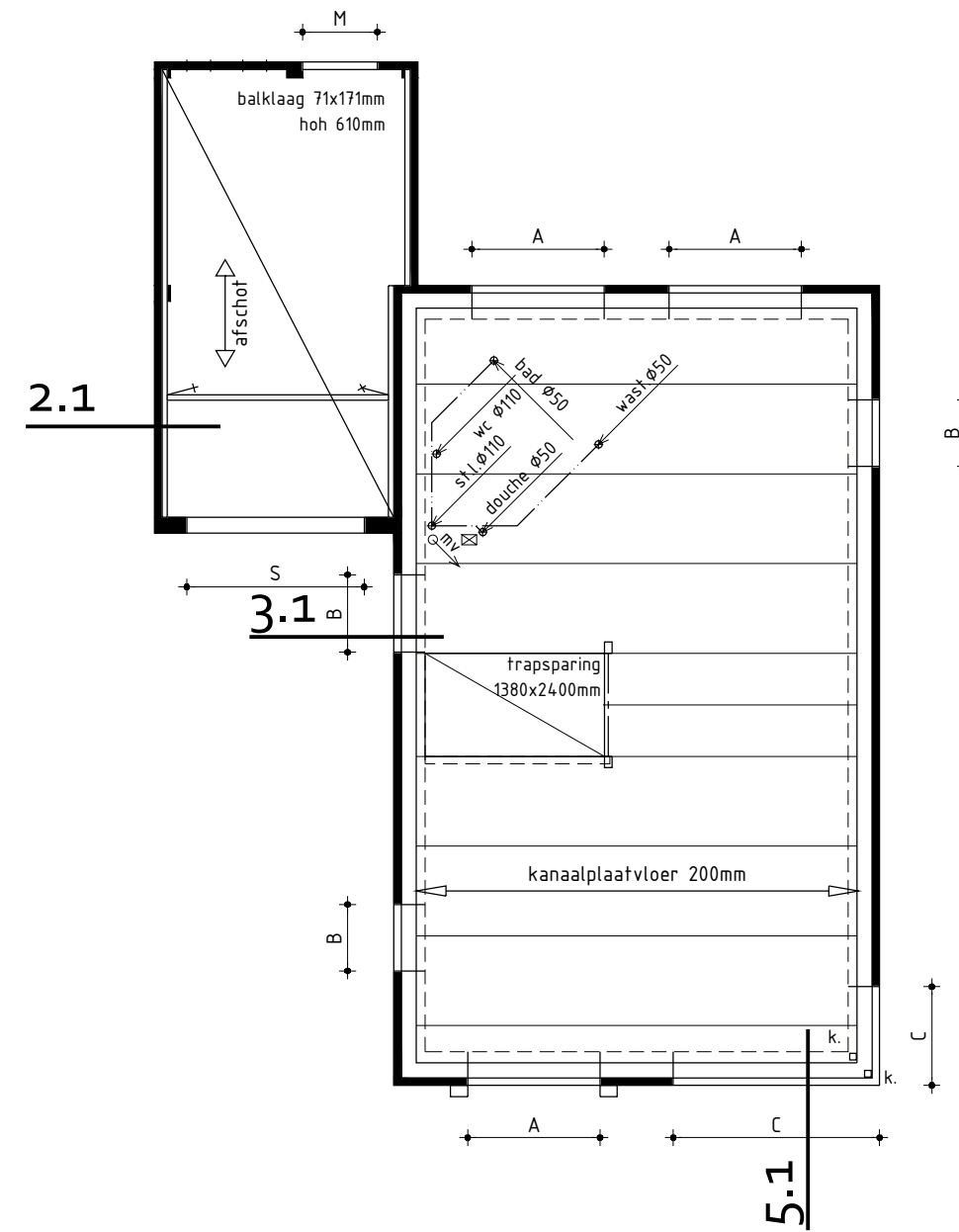
v.z.v. vloerverwarming
