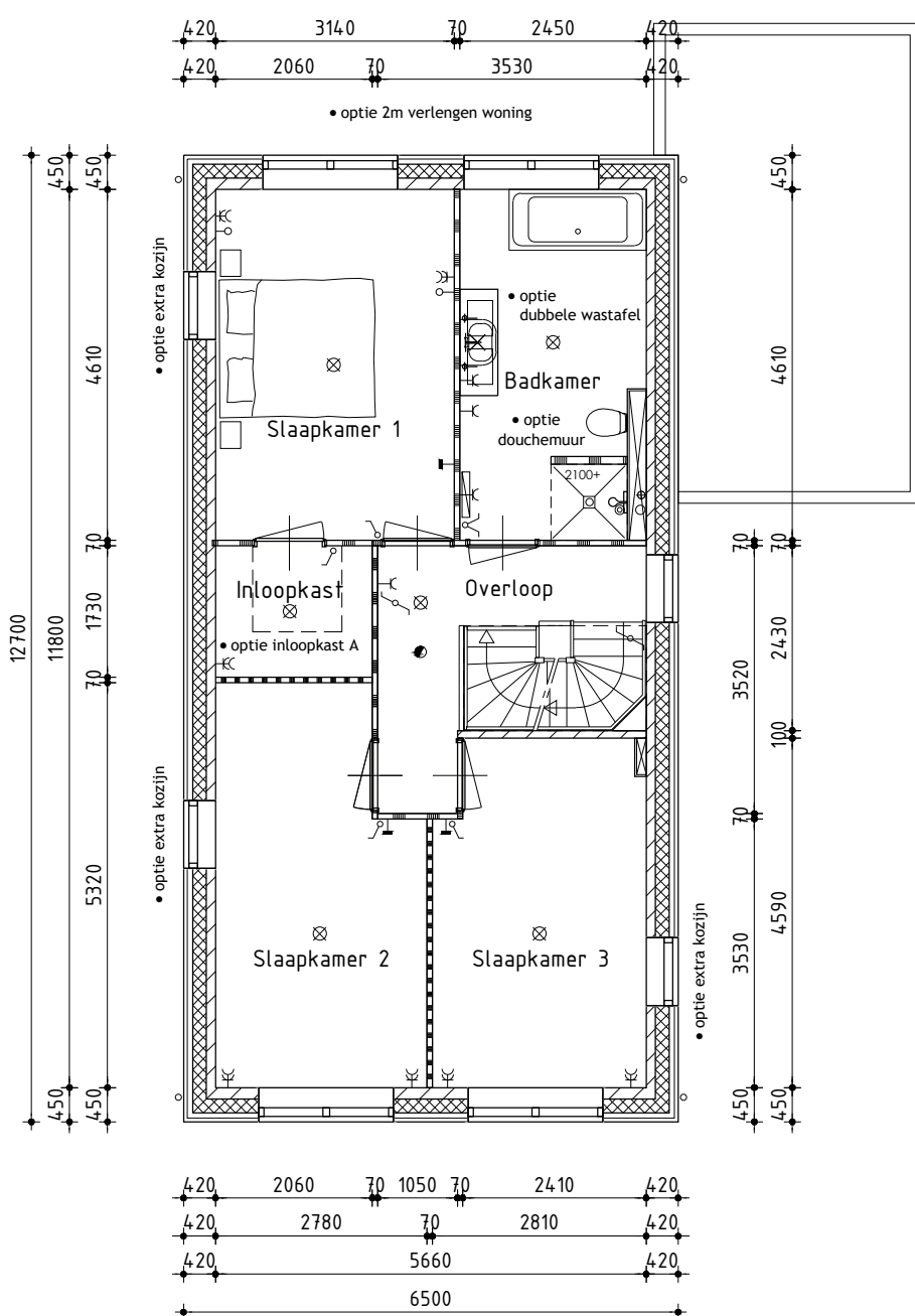
1ste Verdieping
