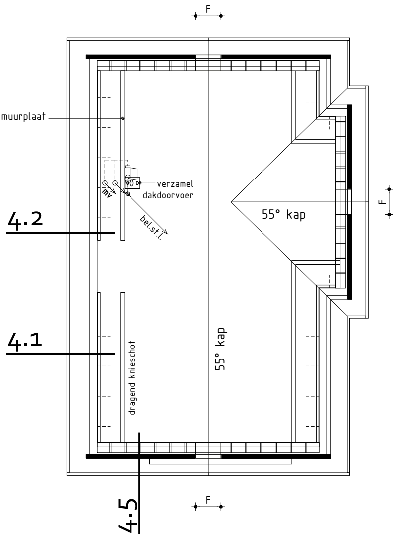
Kapplan
