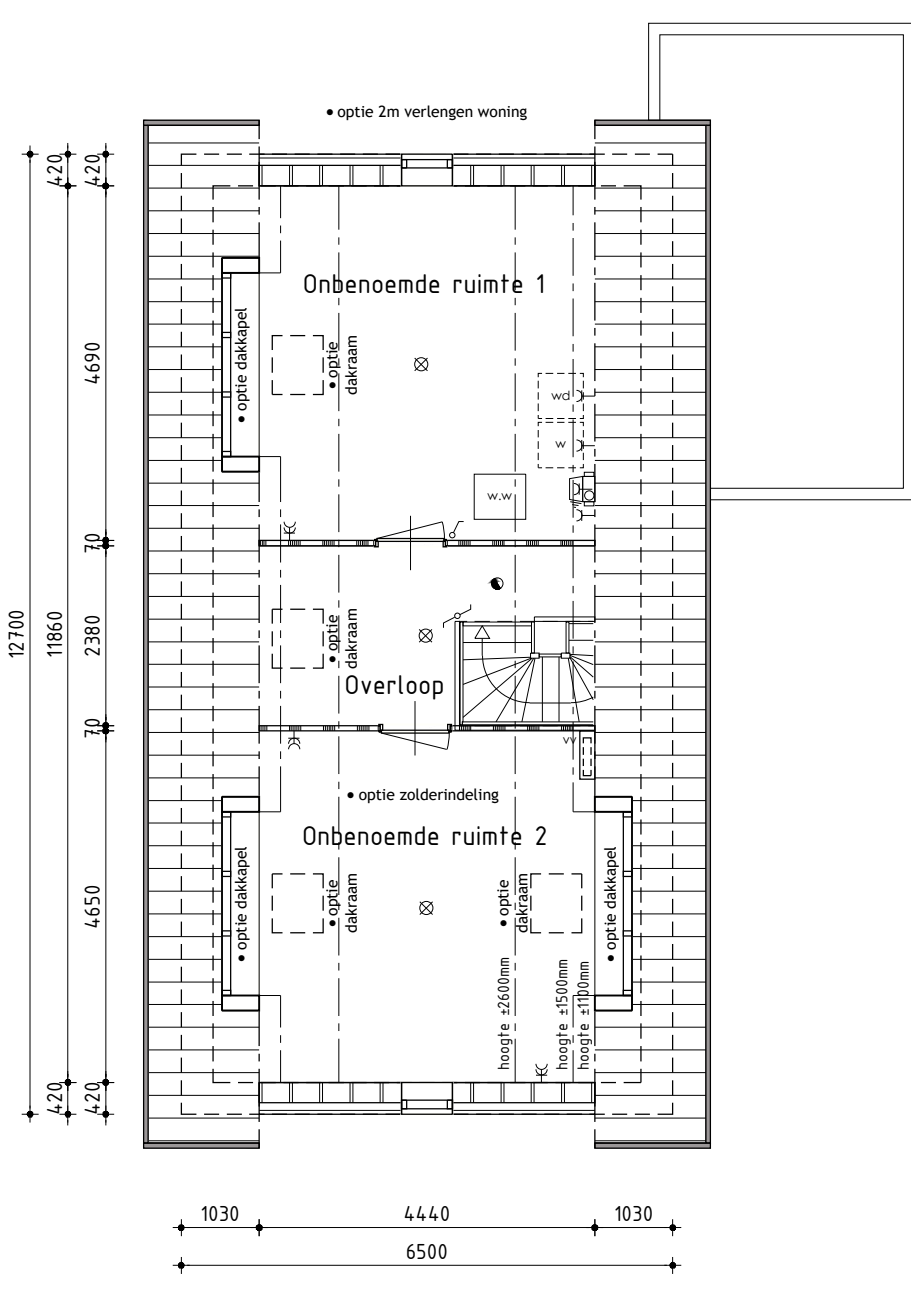
2de Verdieping
