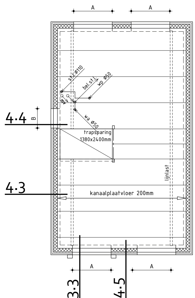
v.z.v. vloerverwarming ALGEMEEN TWEEDE VERDIEPINGSVLOER
