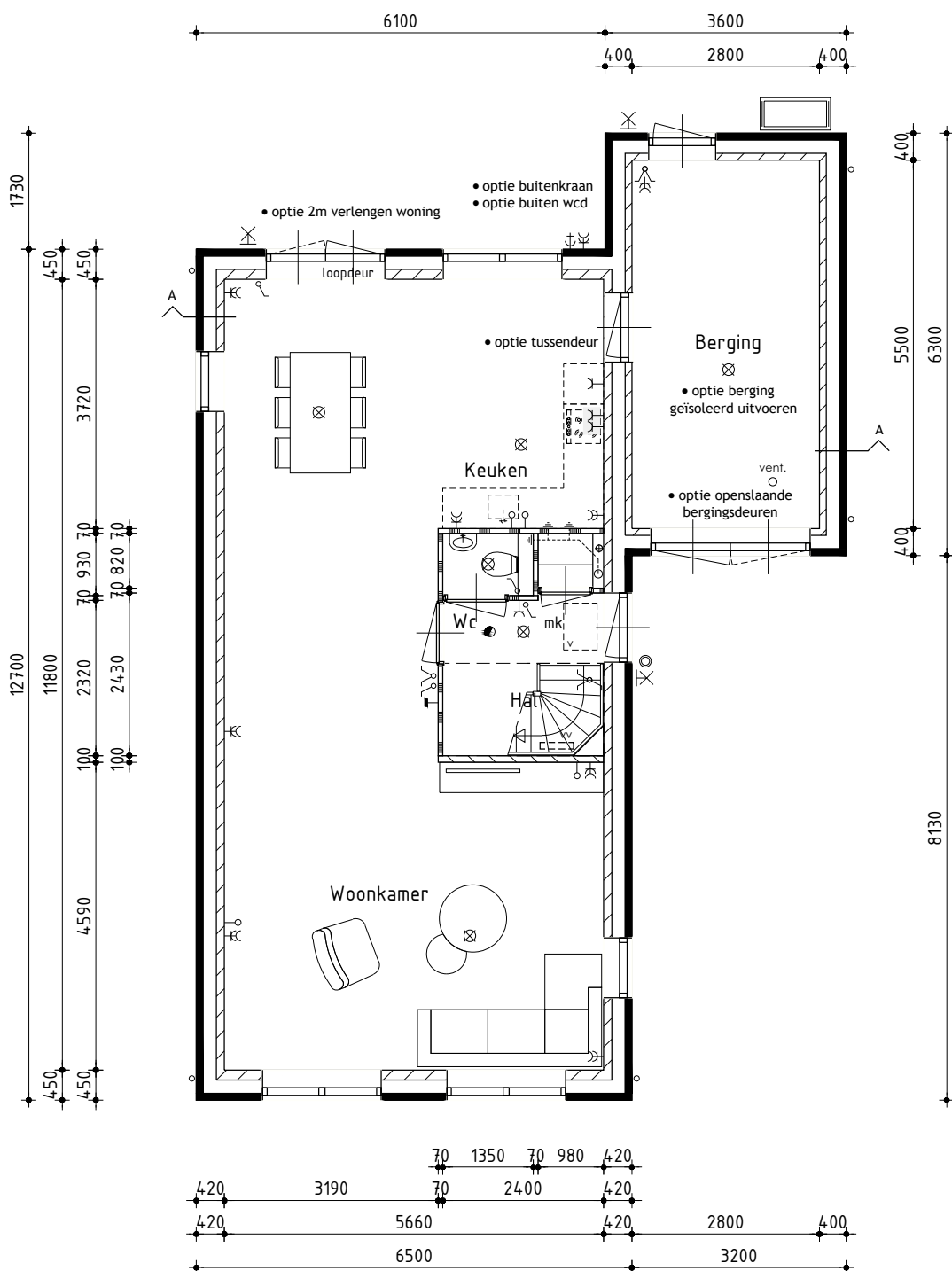
Begane grond
