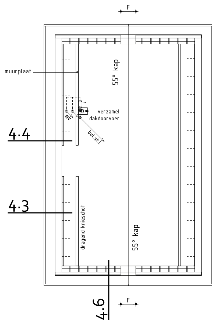
ALGEMEEN KAPPLAN
