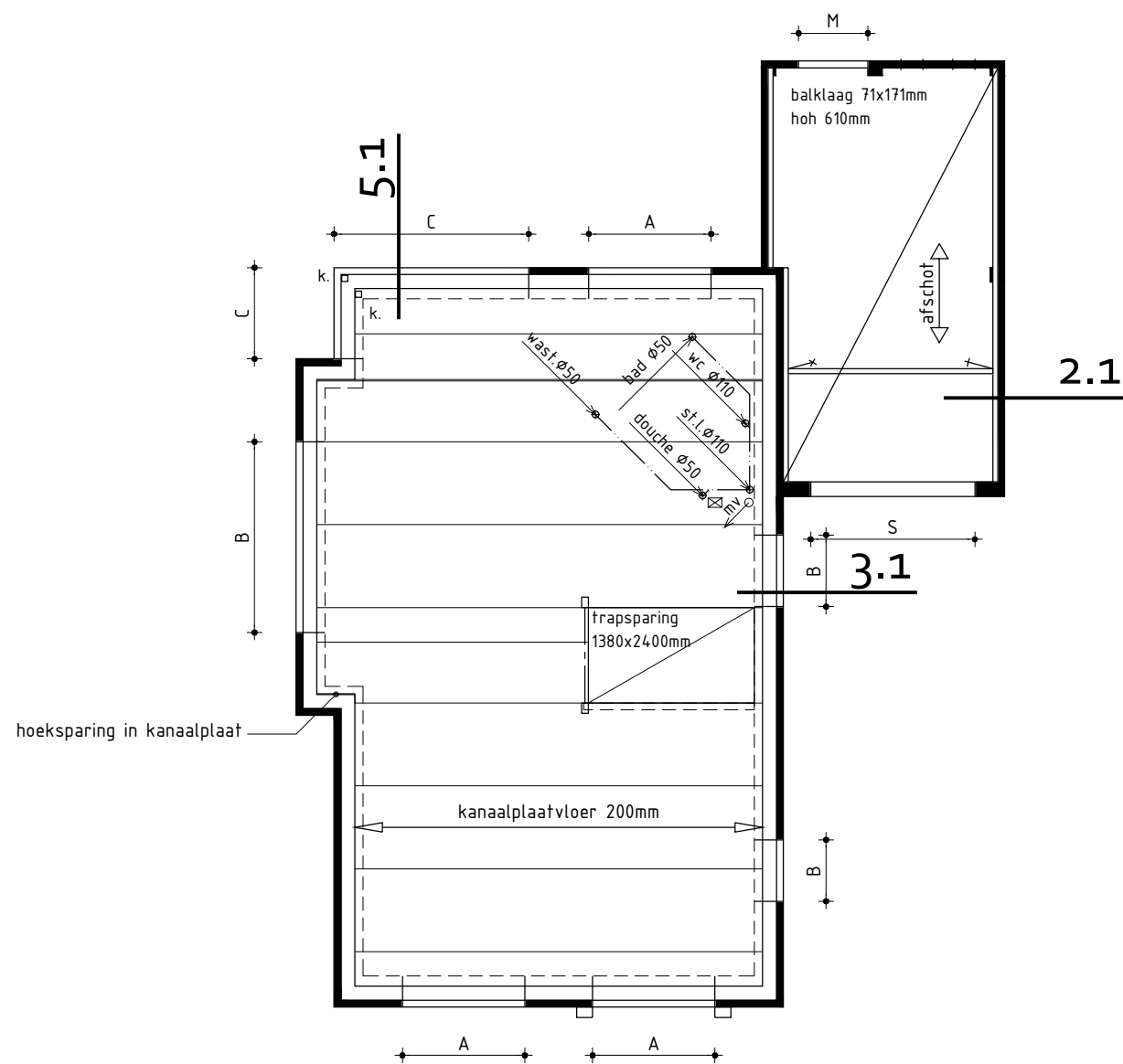
v.z.v. vloerverwarming
