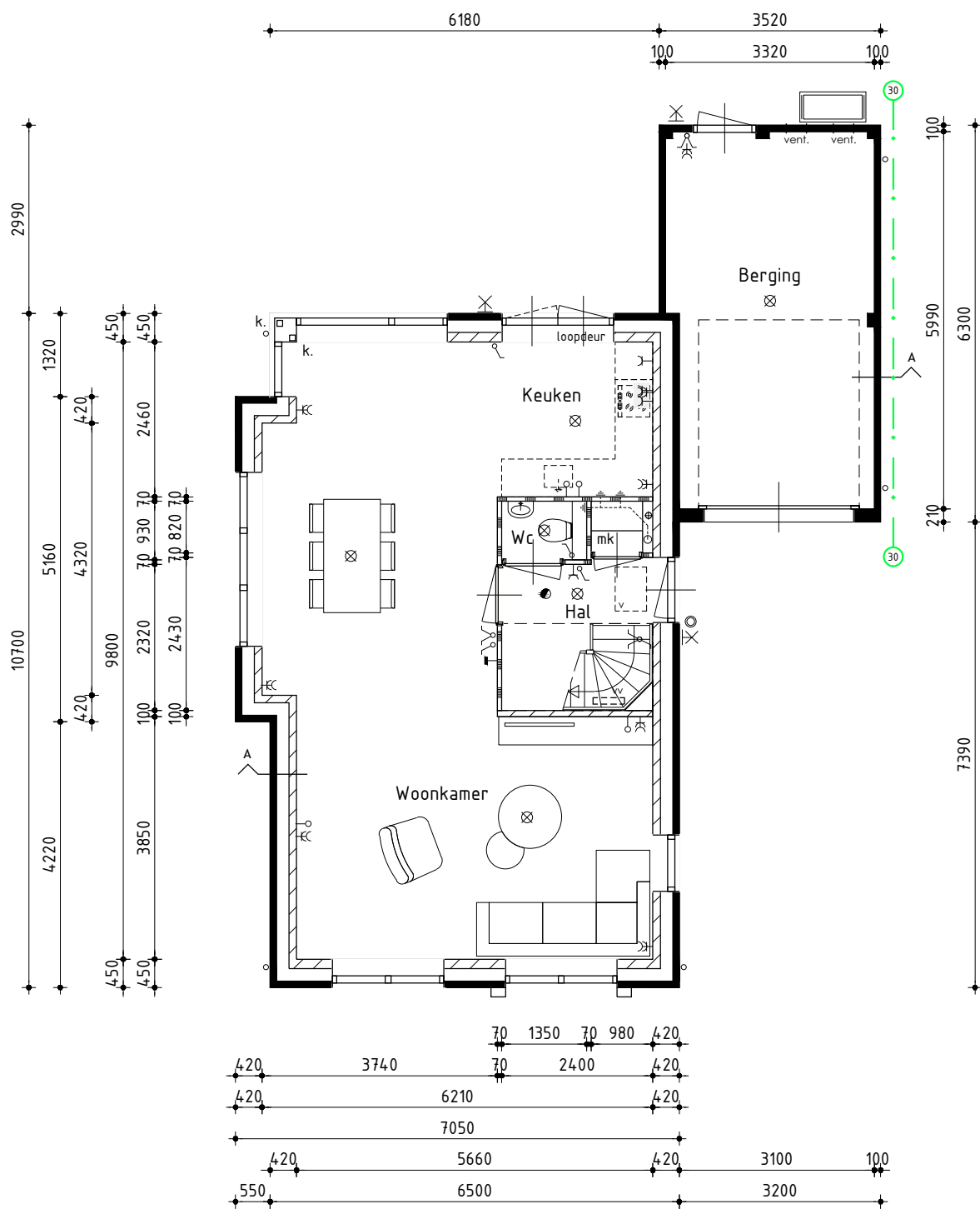
Begane grond
