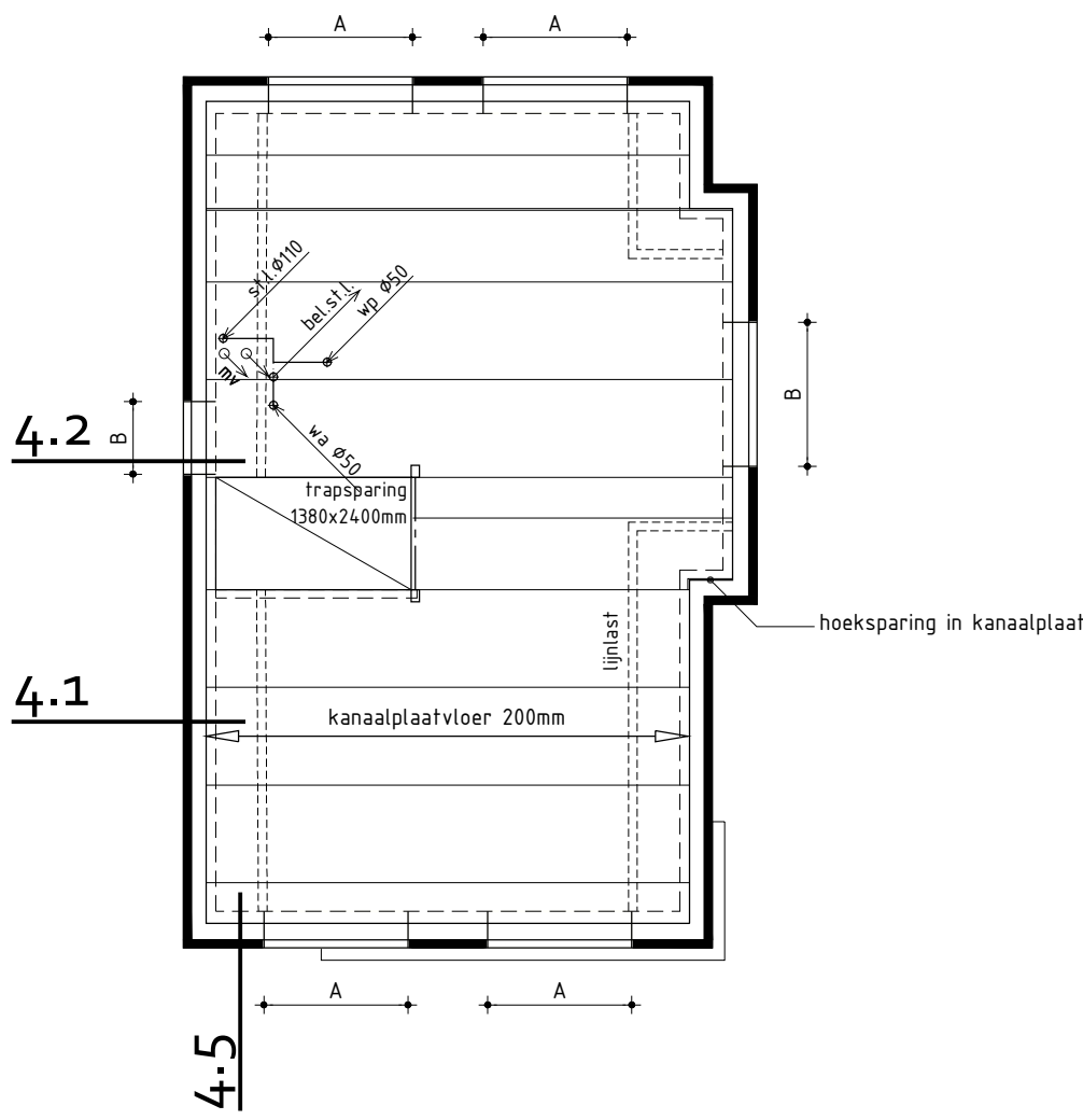
2de Verdiepingsvloer
