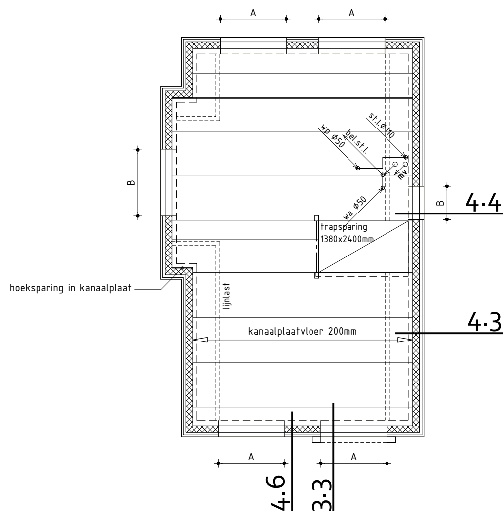
v.z.v. vloerverwarming
