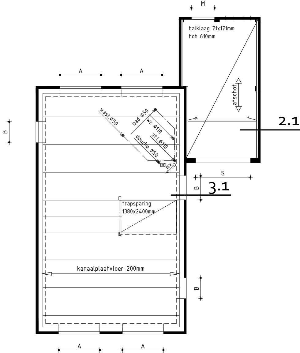
1ste Verdiepingsvloer
