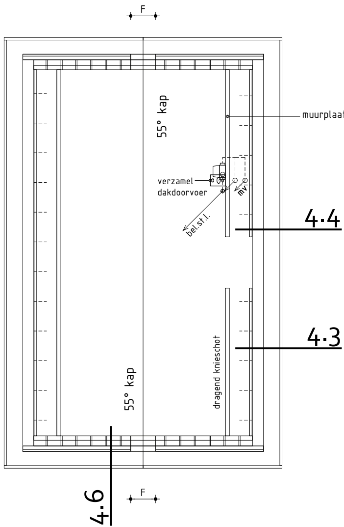
Kapplan
