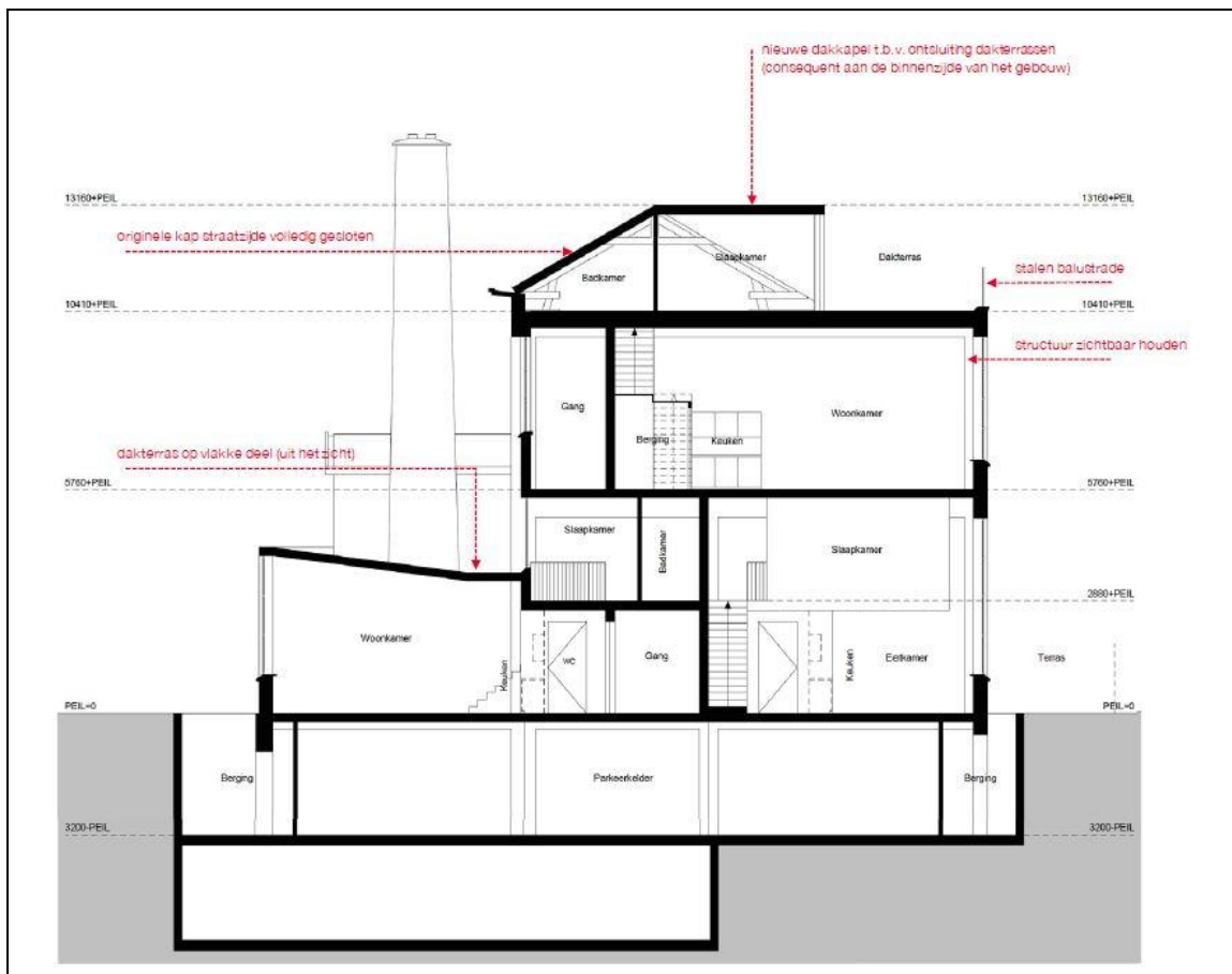
Figuur 10. Een doorsnede van de publiekshal met de geplande wijzigingen aan het monumentale pand de Kerkbrink 16 (bron: Ten Brinke Vastgoed ontvangen op 13-02-2018).
