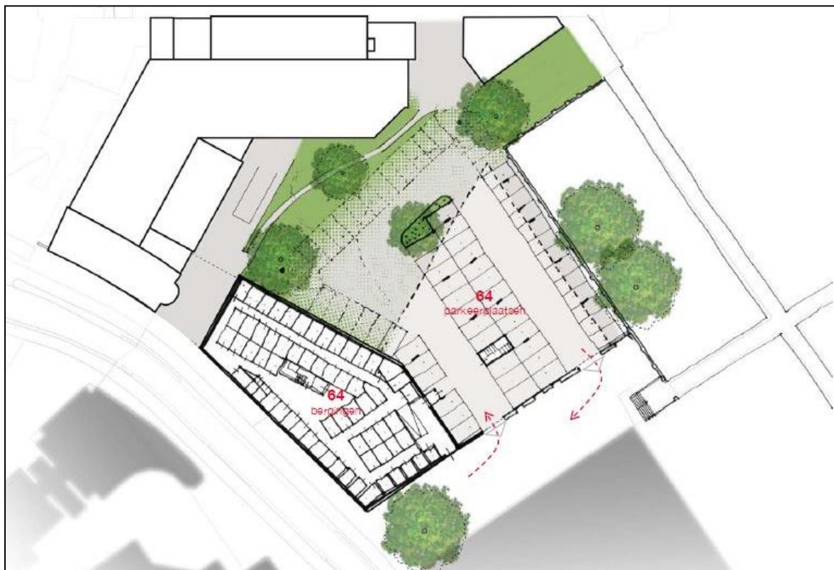
Figuur 9. Nieuwe situatie Oude Torenstraat 1-3 begane grond met bergingen en parkeerplaatsen (bron: Ten Brinke Vastgoed ontvangen op 13-02-2018).
