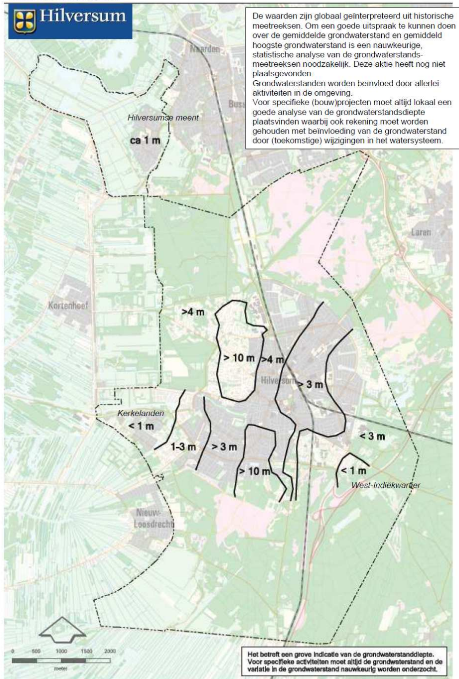
Figuur 1 Minimale grondwaterstandsdiepte Hilversum, globaal geïnterpreteerd, situatie 2011
