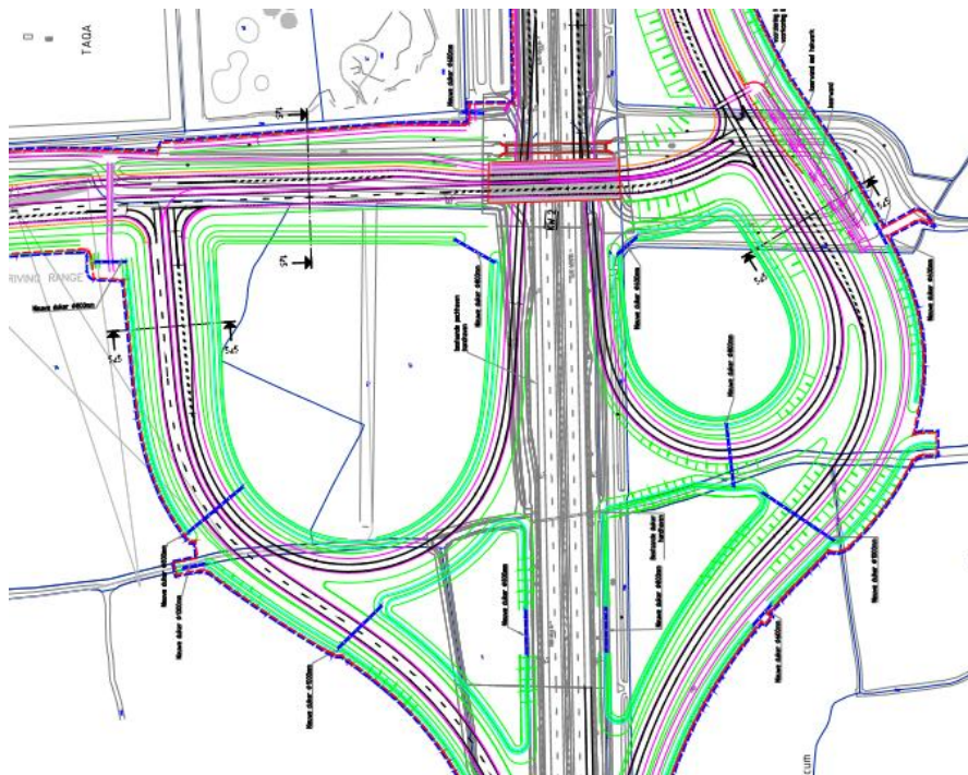
Figuur 10: Situatie met kopsloten en het oplossen daarvan door middel van duikers (blauwe lijn = verbinden watergang middels een duiker)
