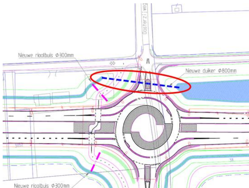
Figuur 12: Locaties van de stuw. Locatie van de stuw is gebaseerd op het waterstructuurplan aangeleverd door Sweco. Stuw wordt ten noordwesten van de turbo rotonde geplaatst.
