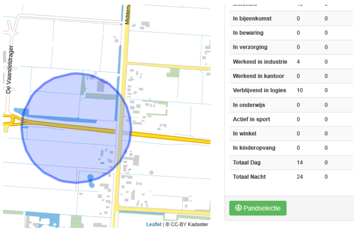
Afbeelding 1: N194 met schadecirkel 200 m. (1% letaal)
