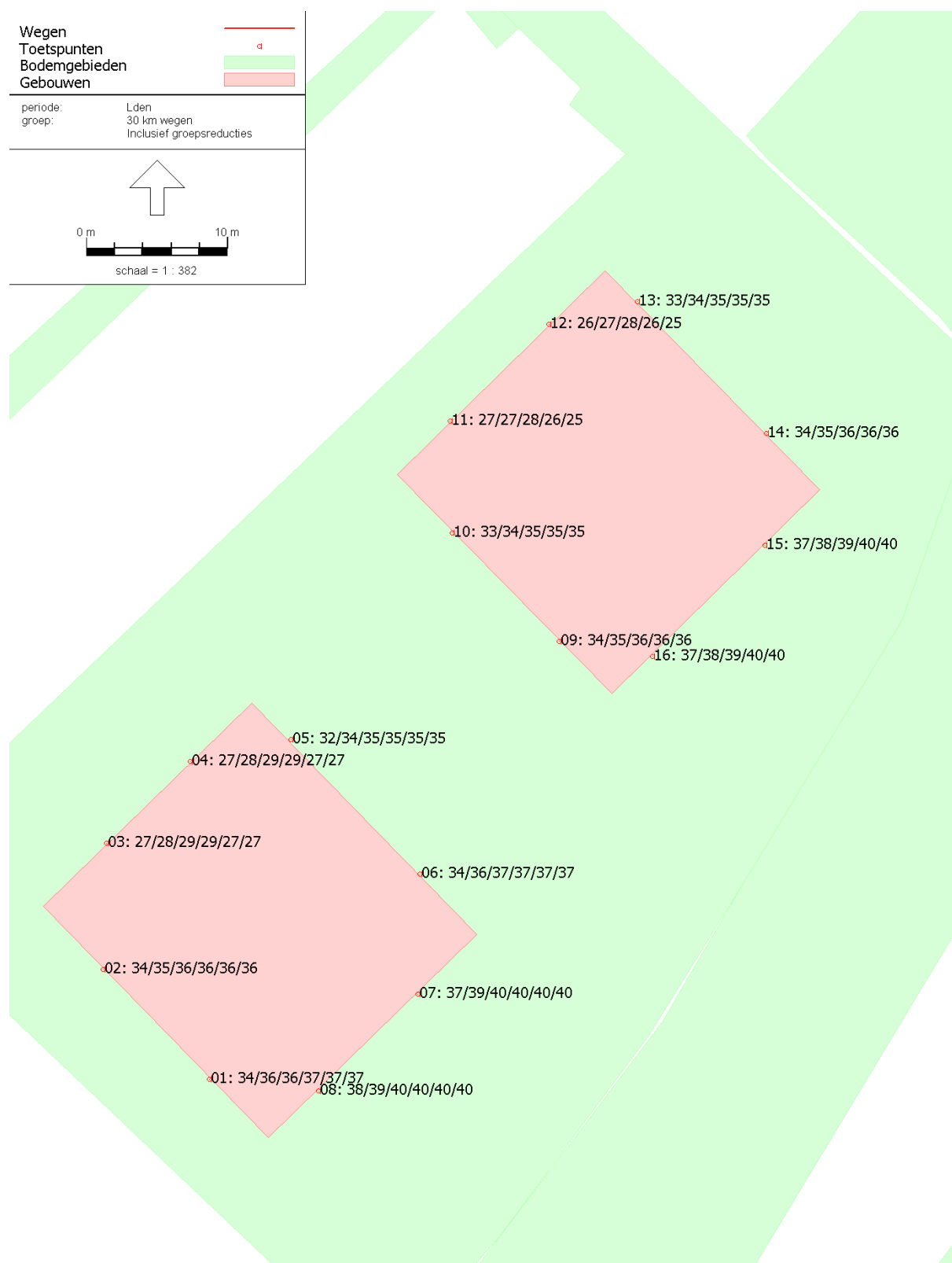
Figuur 5-2 Geluidbelasting 30 km-wegen 2030 inclusief 5 dB aftrek artikel 110 Wgh
