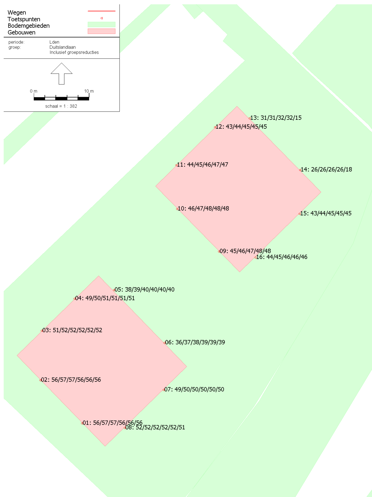
Figuur 5-1 Geluidbelasting Duitslandlaan 2030 inclusief 5 dB aftrek artikel 110 Wgh
