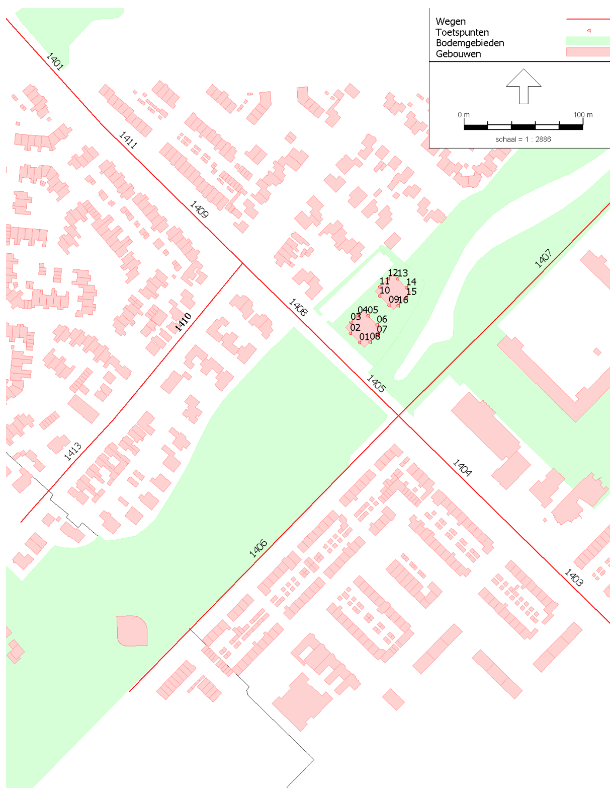
Figuur 4-1 Rekenmodel
