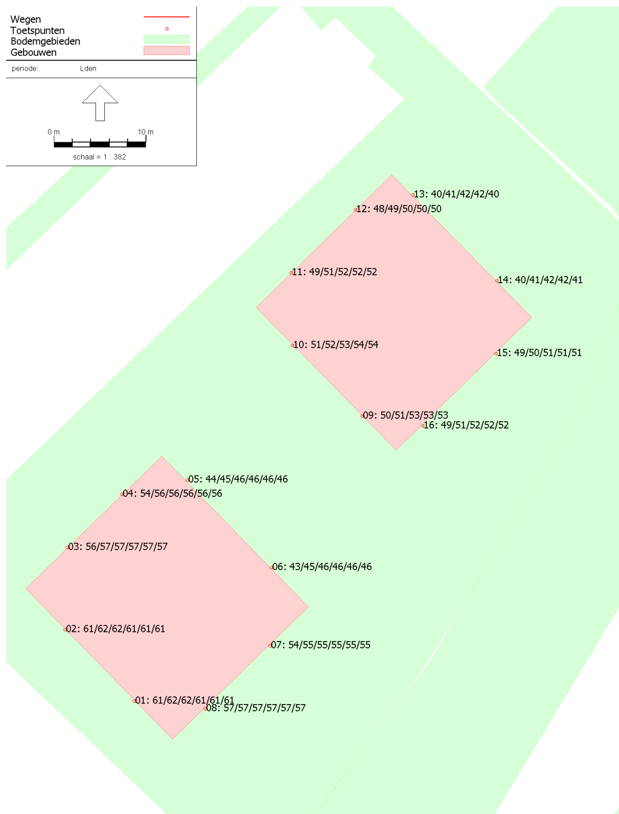
Figuur 5-3 Gecumuleerde geluidbelasting inclusief 0 dB aftrek artikel 110 Wgh
