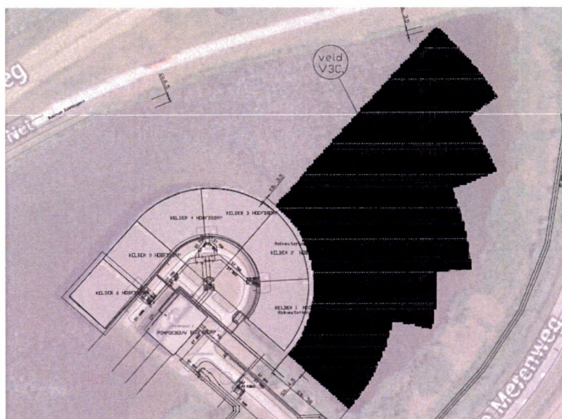
De gewenste situering van de drijvende zonnepanelen in het waterbassin
