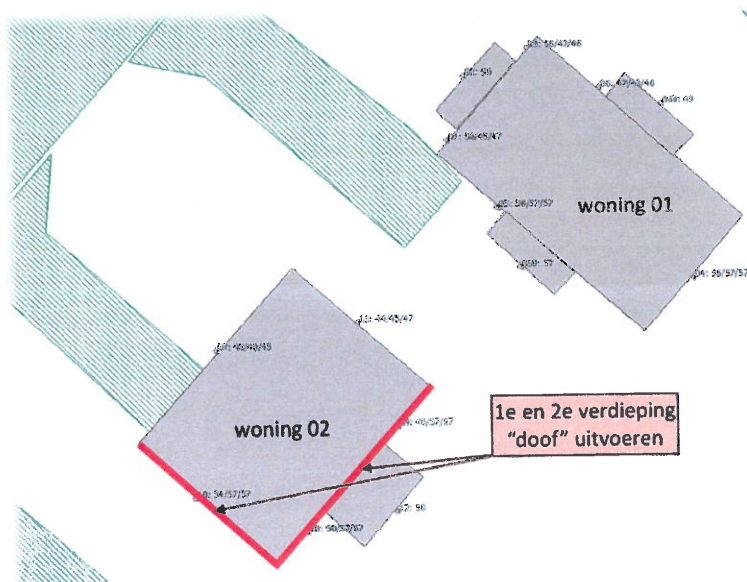
Afbeelding 2.1: Opgegeven geluidbelastingen t.g.v. industrielaawaai (bron ODNZKG)
