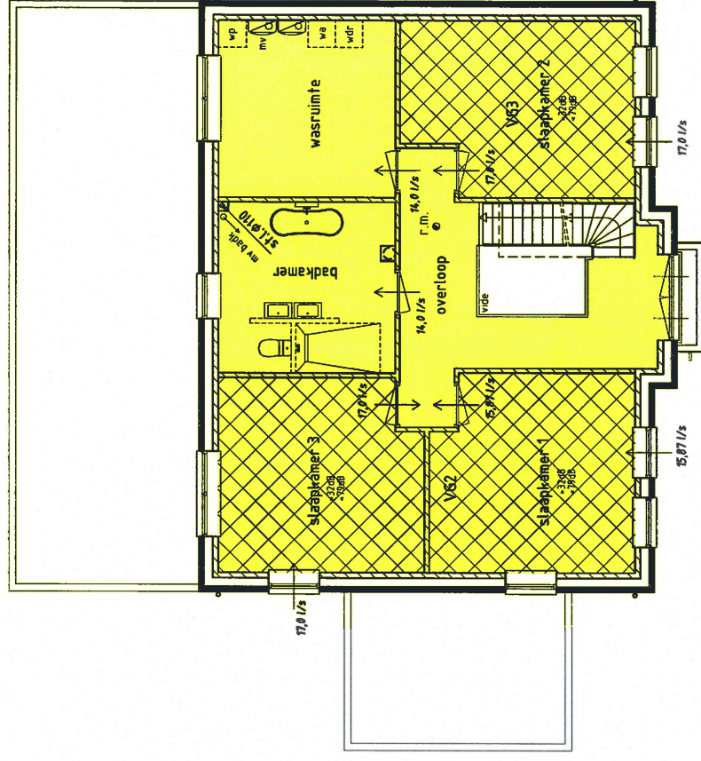
1e Verdieping
