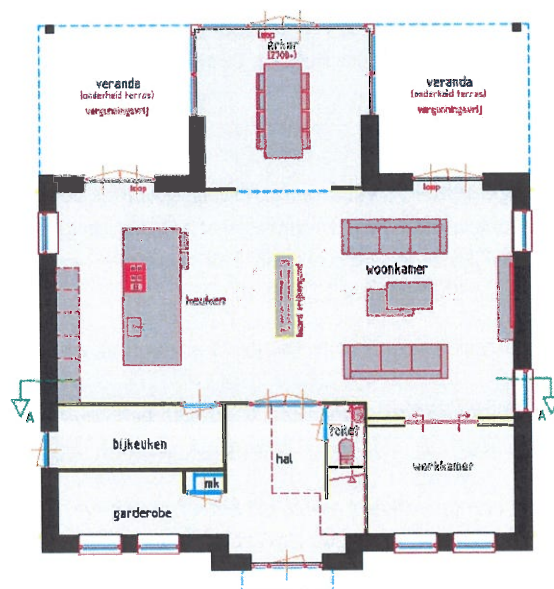
Afbeelding 3.2: Ontwerp woning kavel B – niet op schaal (beganegrand)
