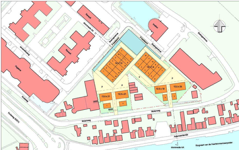
Eindplan: situatie met programma (26 bedrijfswoningen + 4 bedrijfswoningen)
