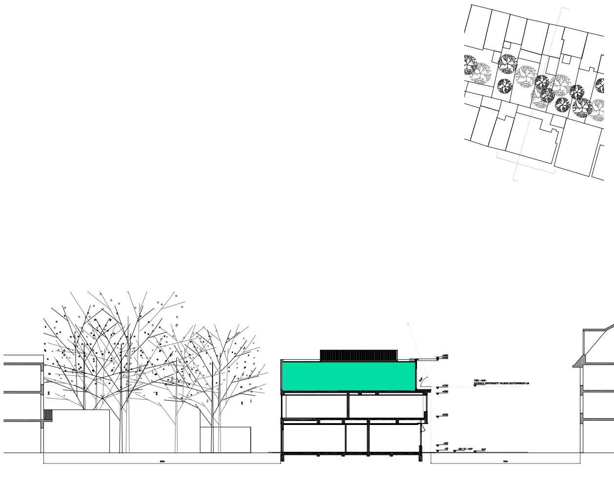
Figuur 10 Doorsnede
