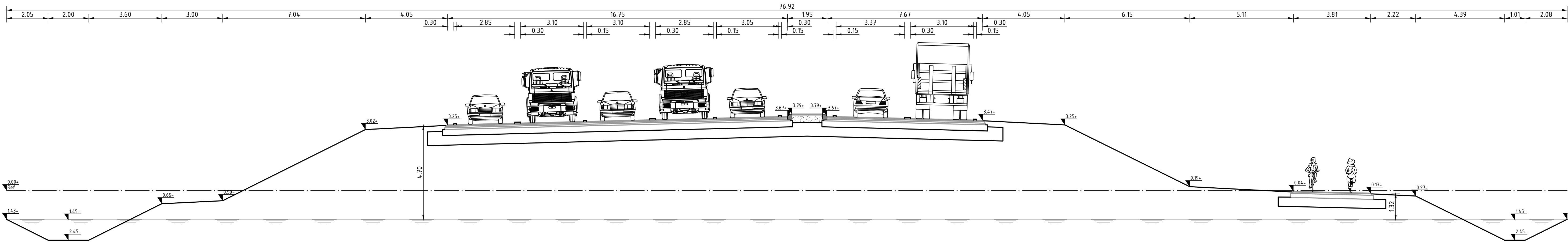
PROFIEL DERDE ONTSLUITINGSWEG 0075
