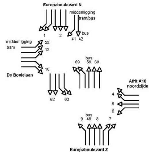
Schematisch overzicht: aanbevolen profielconfiguratie na toetsing
