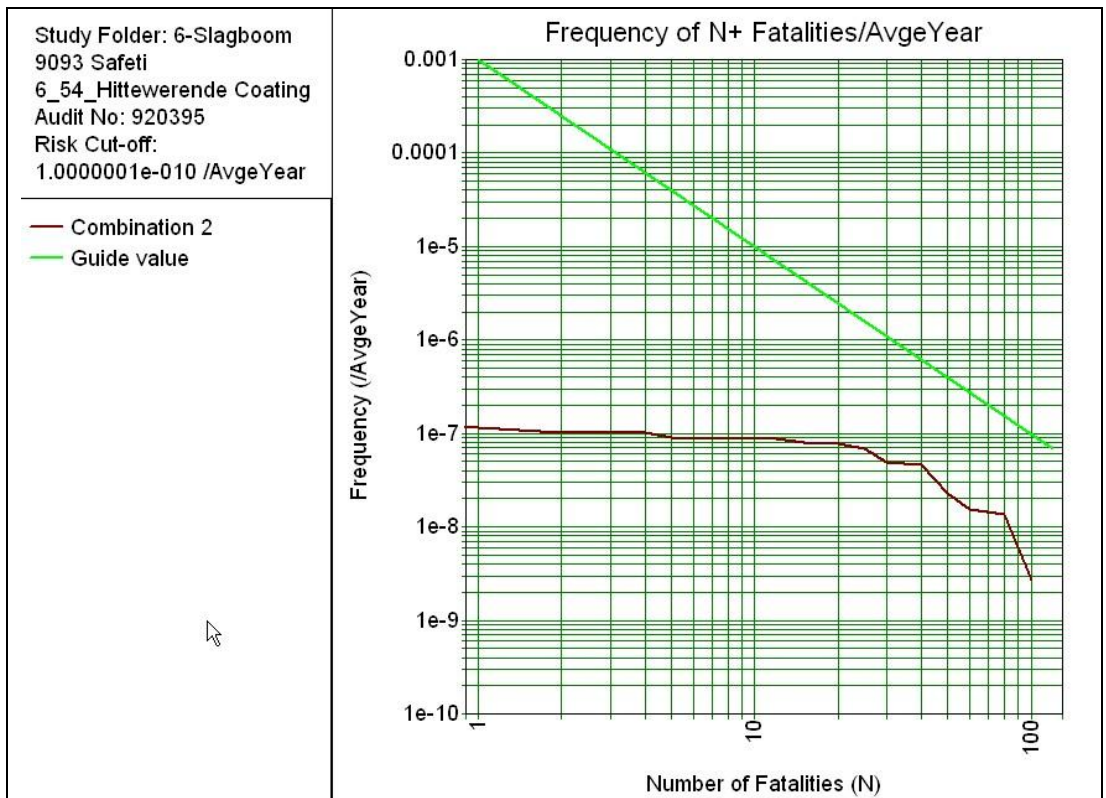
Figuur 2: Berekening van het groepsrisico met LPG convenant maatregel hittewerende coating
