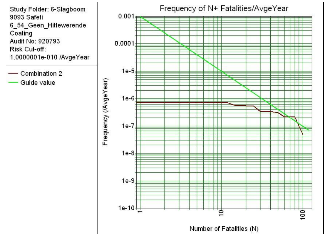
Figuur 1: Berekening van het groepsrisico zonder LPG convenant maatregel hittewerende coating
