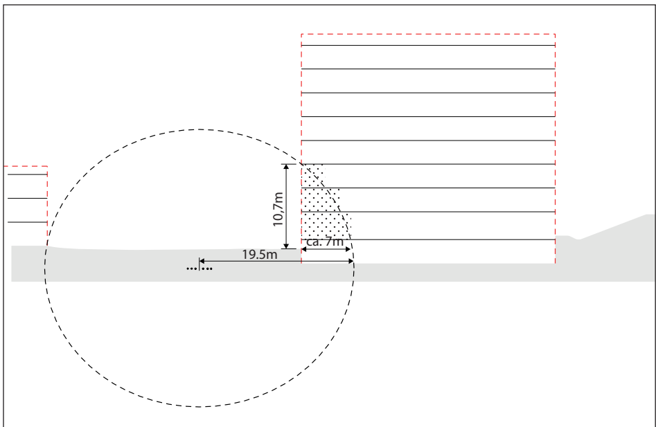
DOORSNEDE C-C
