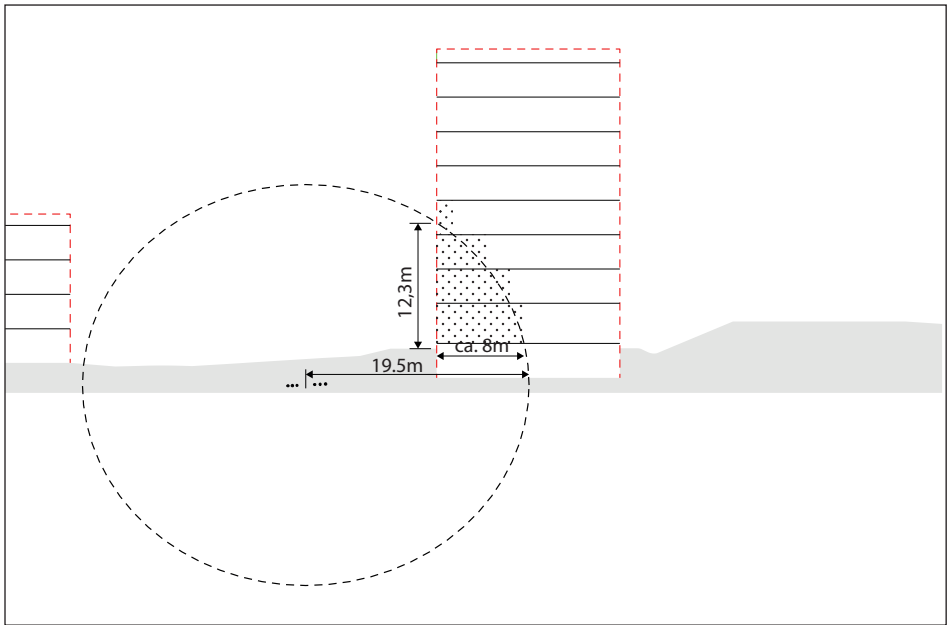
DOORSNEDE A-A
